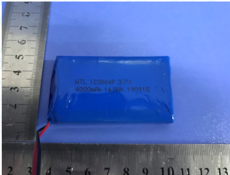
Photo 13 Battery Parameter
