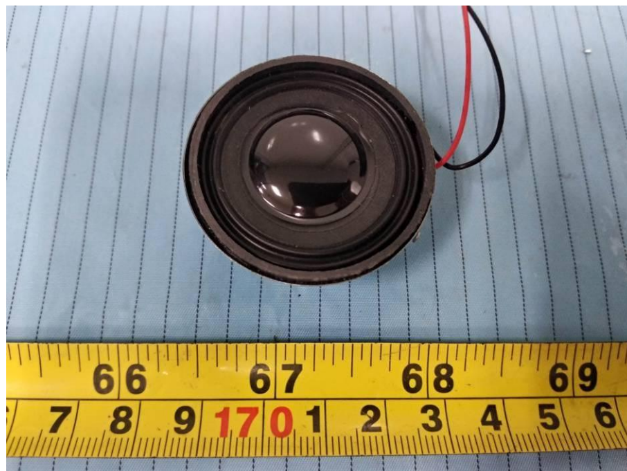
EUT –Horn Top View
