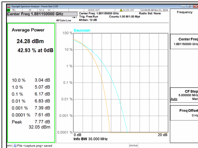
2C / 20+15MHz / Mid CH / QPSK
