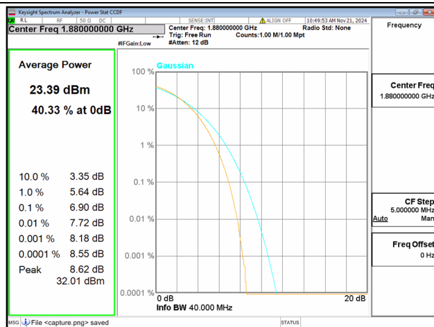
2C / 20+20MHz / Mid CH / 16QAM
