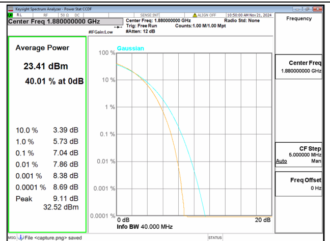
2C / 20+20MHz / Mid CH / 64QAM
