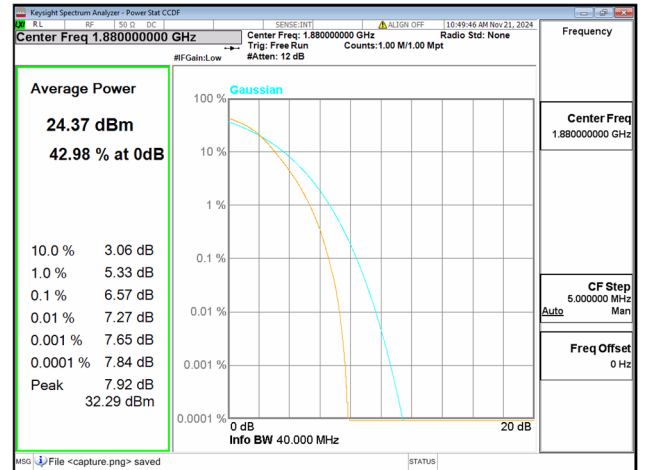
2C / 20+20MHz / Mid CH / QPSK
