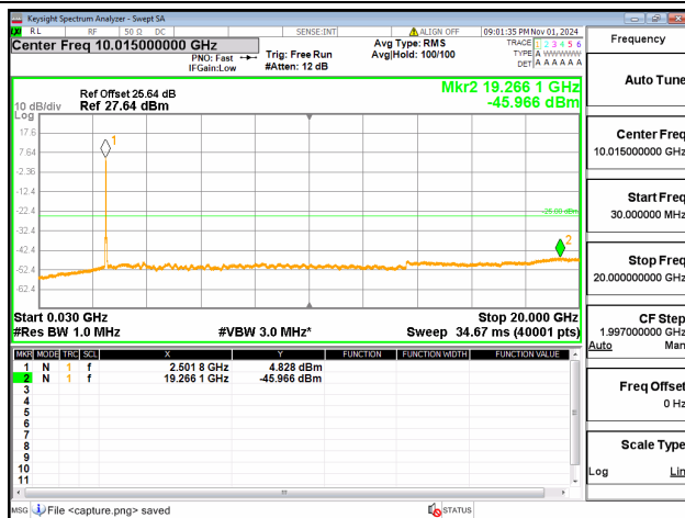
41C-30M-20G / 20+10MHz / QPSK / Low CH / 100@0-50@0
