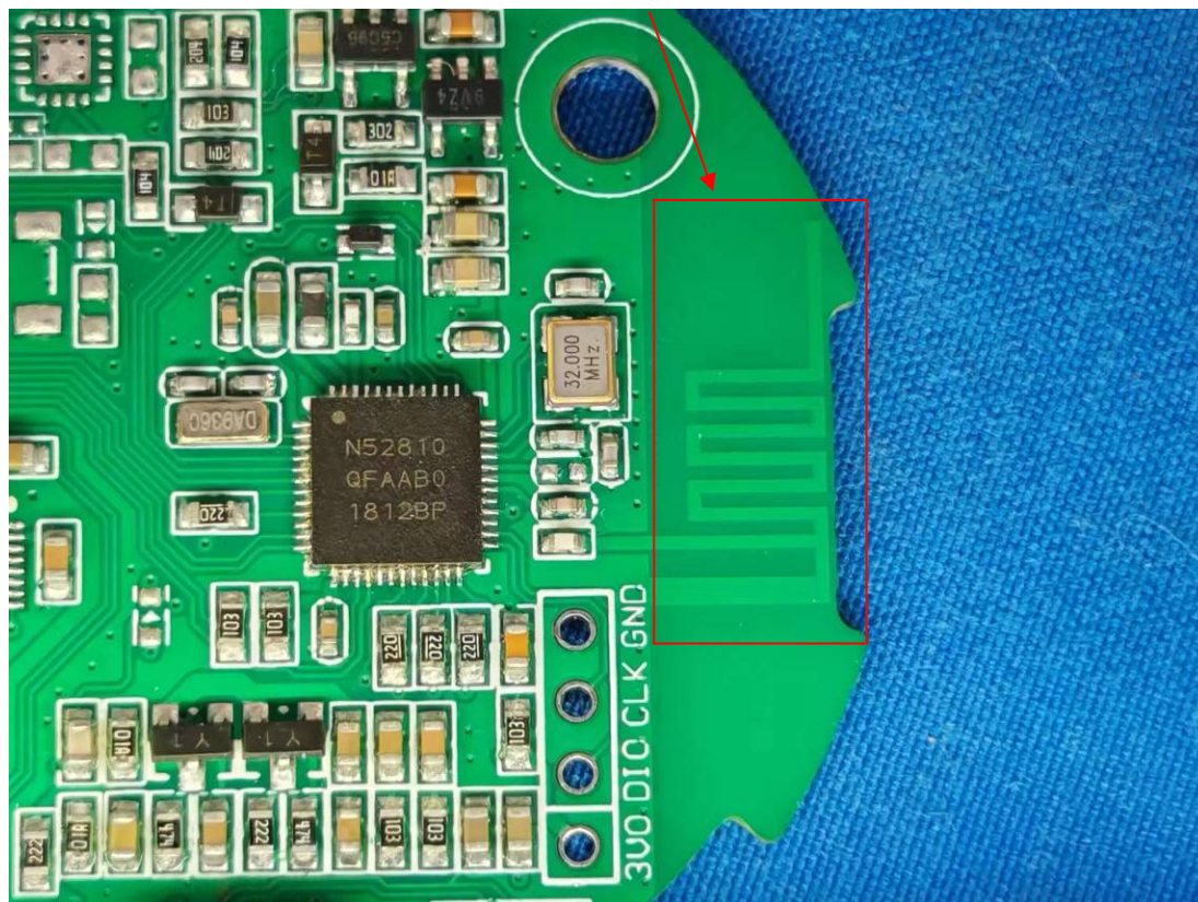
BLE Antenna
