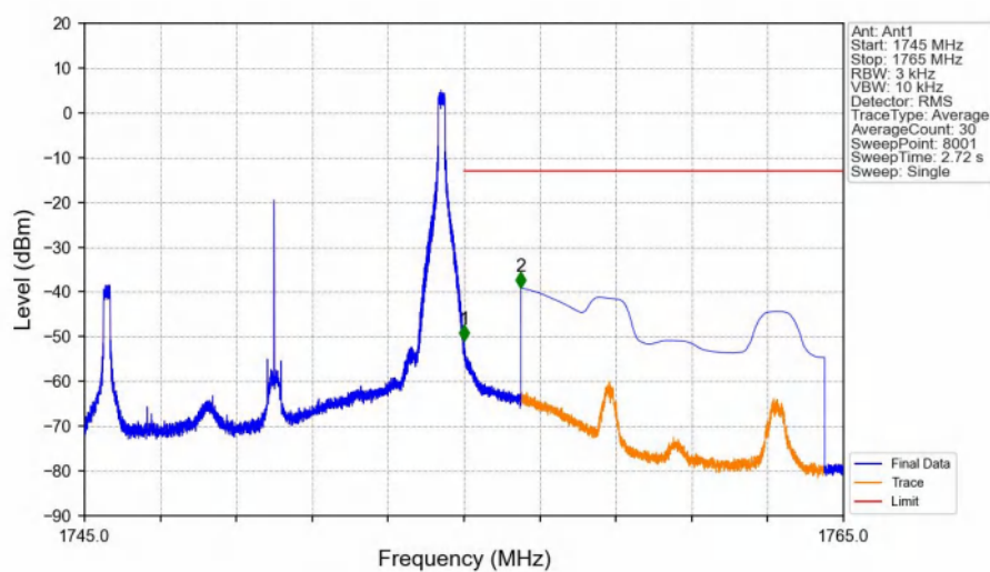
Band4_10MHz_QPSK_HCH_1750MHz_RB_1_49_NTNV
