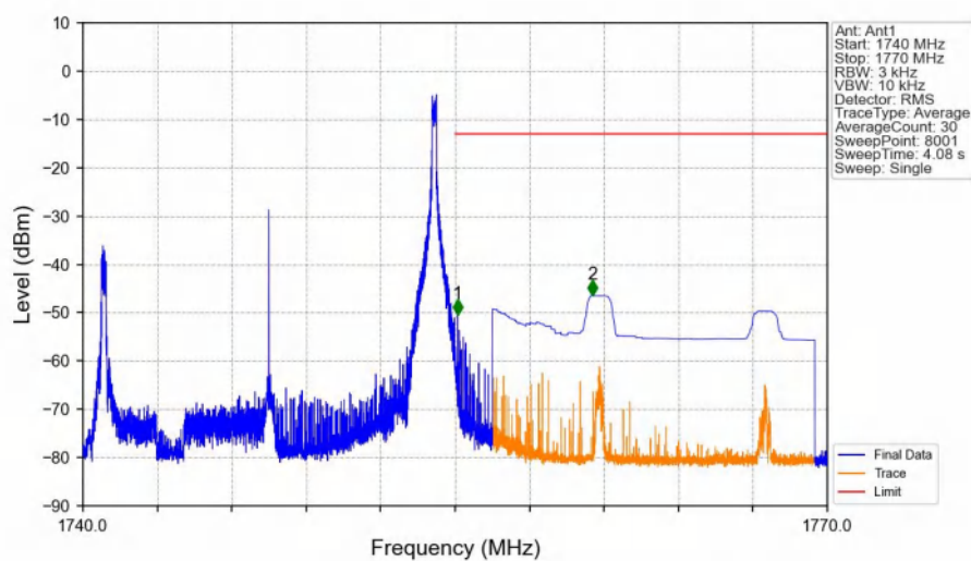
Band4_15MHz_QPSK_HCH_1747.5MHz_RB_1_74_NTNV
