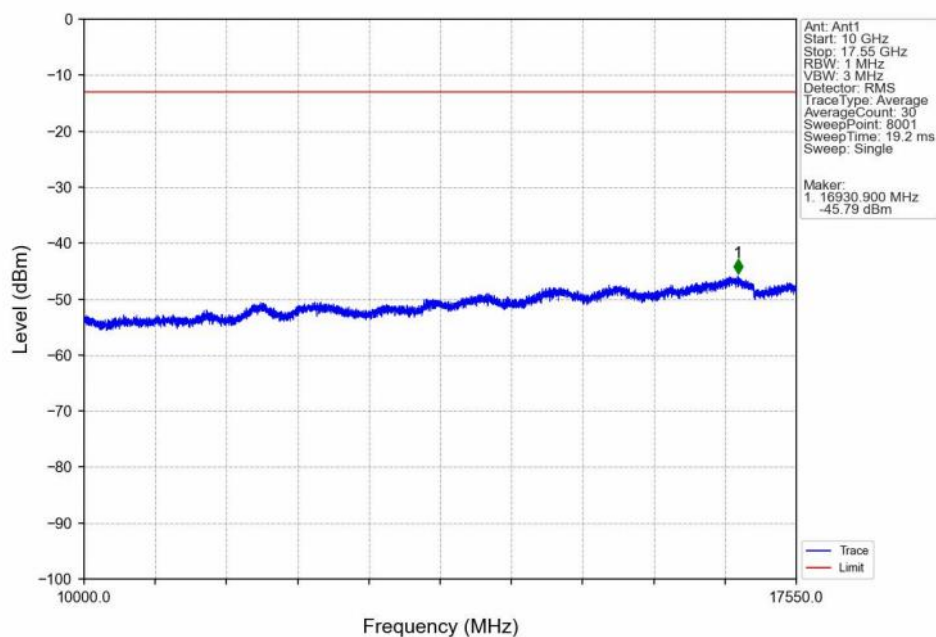
Band4_15MHz_QPSK_HCH_1747.5MHz_RB_1_74_NTNV
