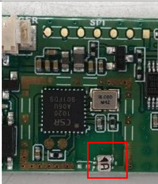
BLE Antenna
