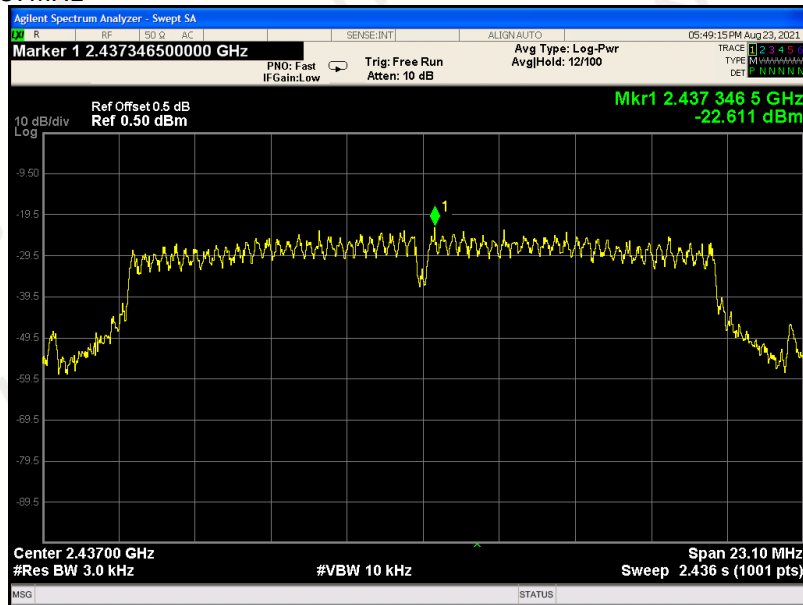
CH6: 2437MHz
