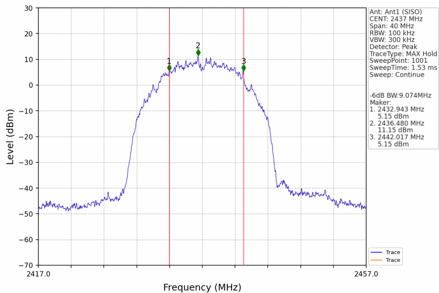
802.11b_MCH_2437MHz_Ant1 (SISO)_NTNV
