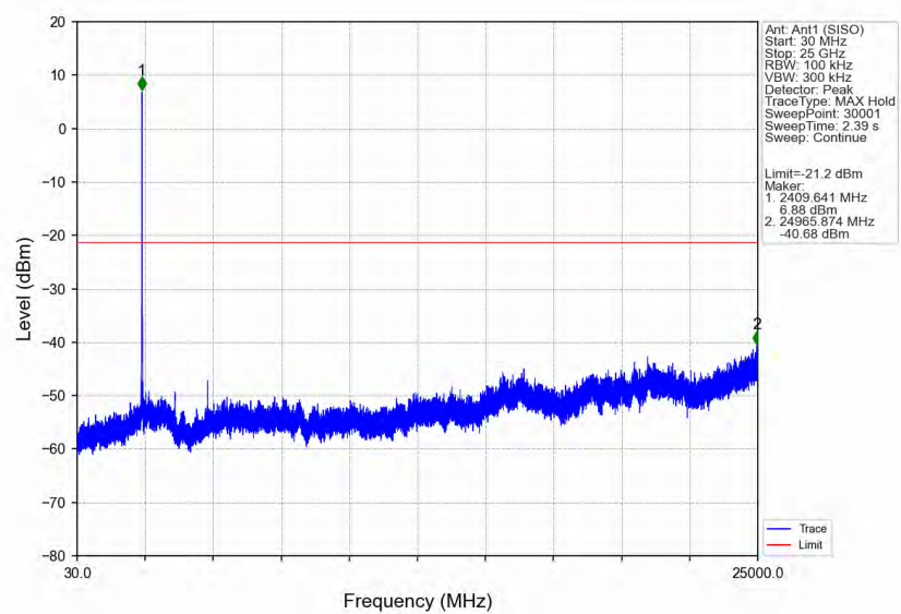
802.11b_LCH_2412MHz_Ant1 (SISO)_NTNV
