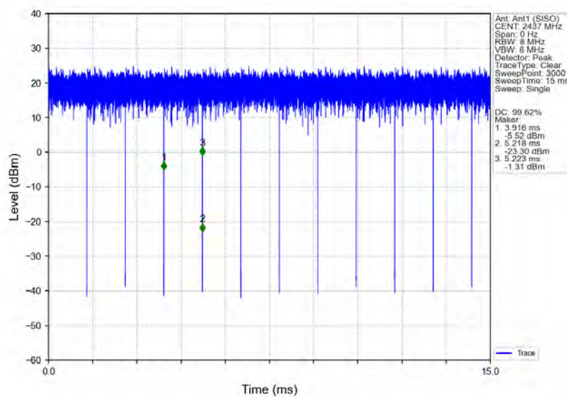
802.11n(HT20)_MCH_2437MHz_Ant1 (SISO)_NTNV
