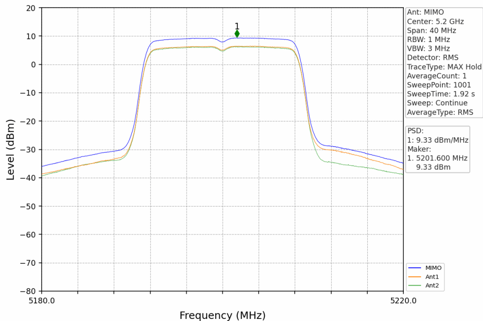
802.11n(HT20)_MCH_5200MHz_MIMO_NTNV
