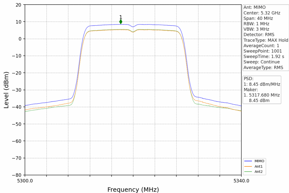
802.11n(HT20)_HCH_5320MHz_MIMO_NTNV
