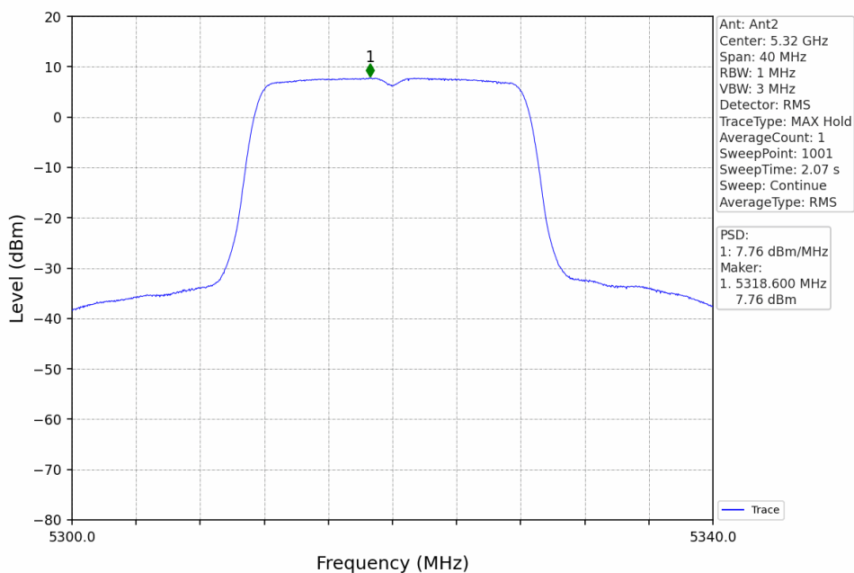
802.11a_HCH_5320MHz_Ant2_NTNV
