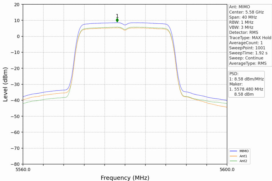
802.11n(HT20)_MCH_5580MHz_MIMO_NTNV
