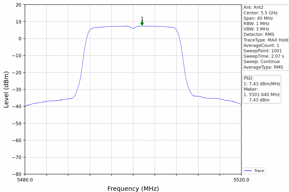
802.11a_LCH_5500MHz_Ant2_NTNV
