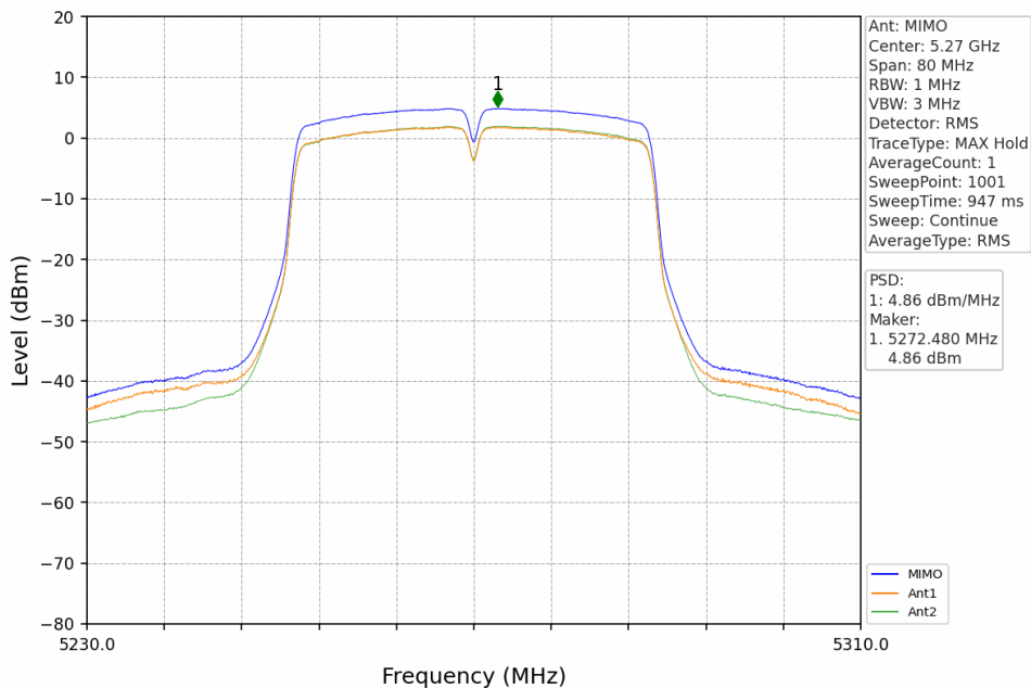
802.11n(HT40)_LCH_5270MHz_MIMO_NTNV
