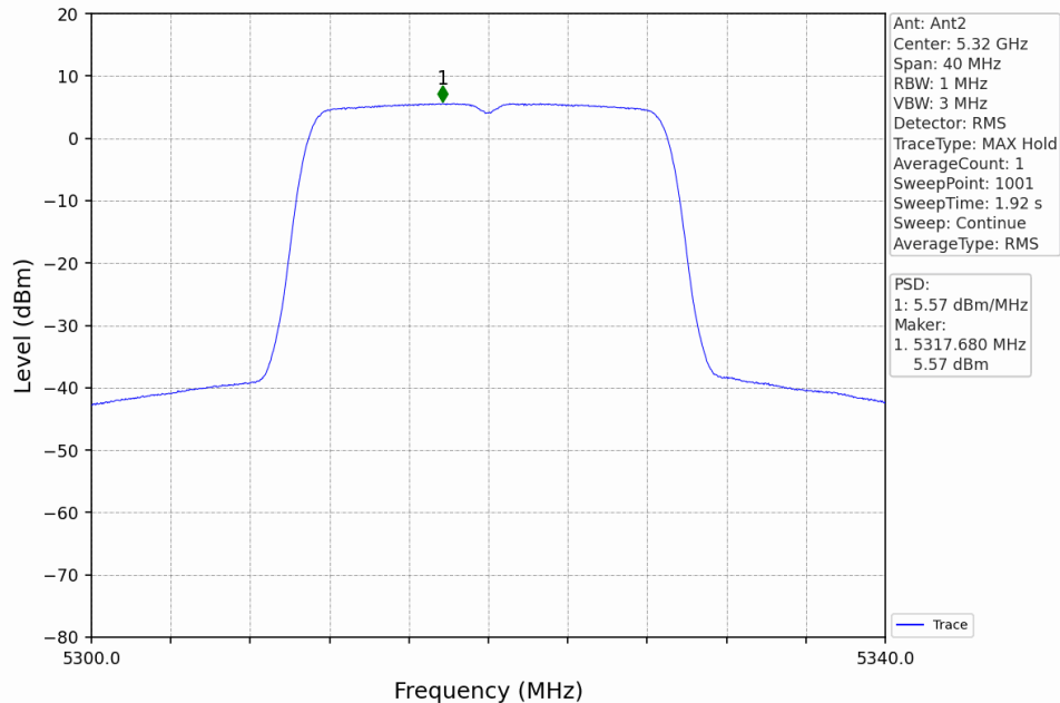
802.11n(HT20)_HCH_5320MHz_MIMO_NTNV
