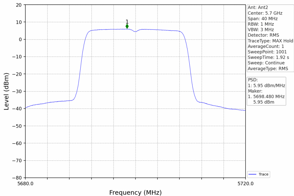
802.11n(HT20)_HCH_5700MHz_Ant2_NTNV
