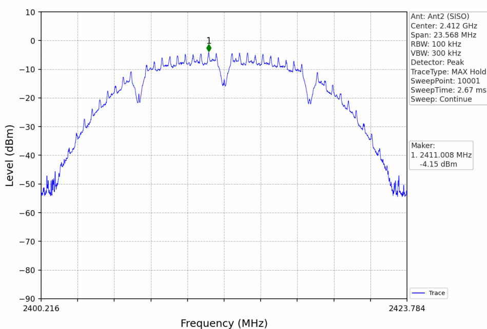
802.11g_LCH_2412MHz_Ant2 (SISO)_NTNV
