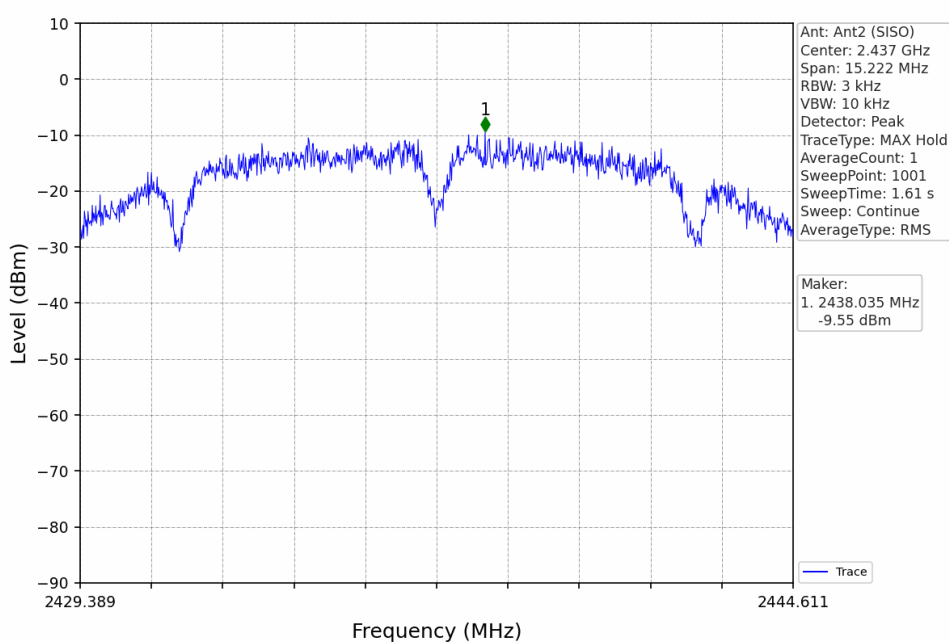
802.11b_MCH_2437MHz_Ant2 (SISO)_NTNV
