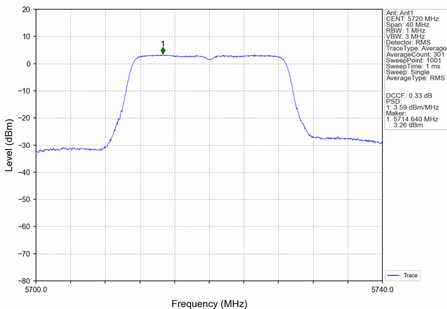
802.11n(HT20)_HCH_5720MHz_Ant1_NTNV
