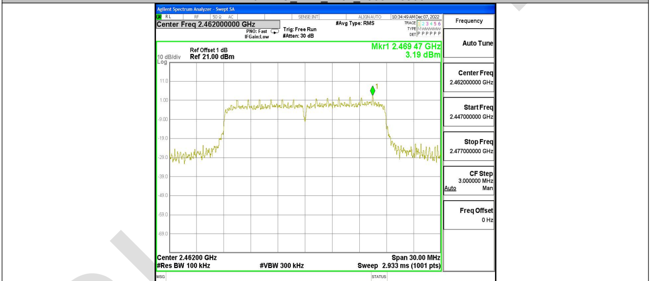
11N20MIMO_Ant2_2462_0~Reference
