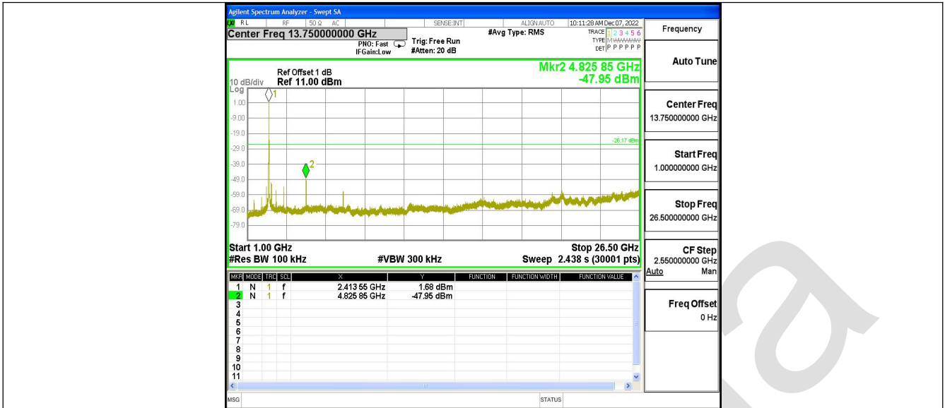
11N20MIMO_Ant1_2412_1000~26500
