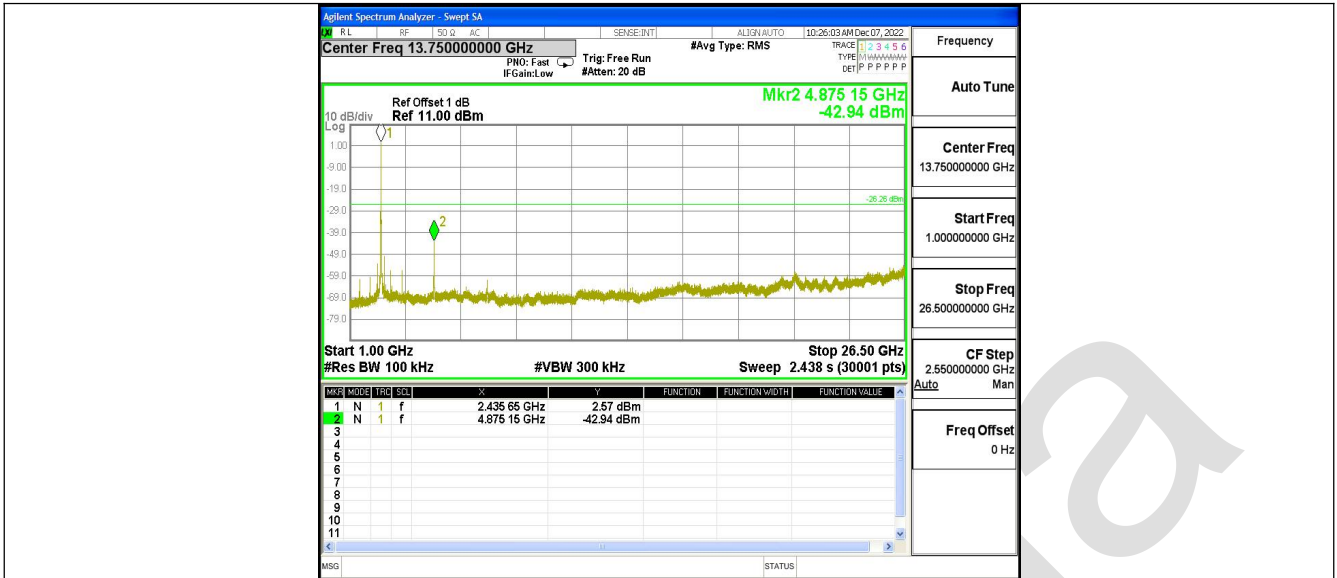
11N20MIMO_Ant1_2437_1000~26500
