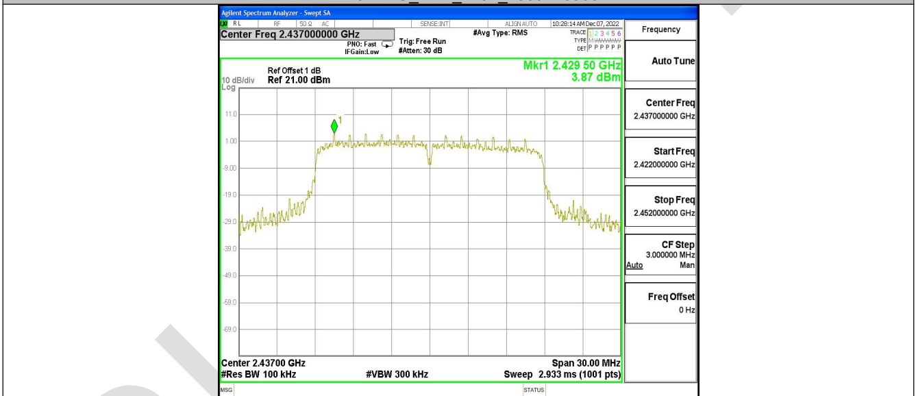
11N20MIMO_Ant2_2437_0~Reference
