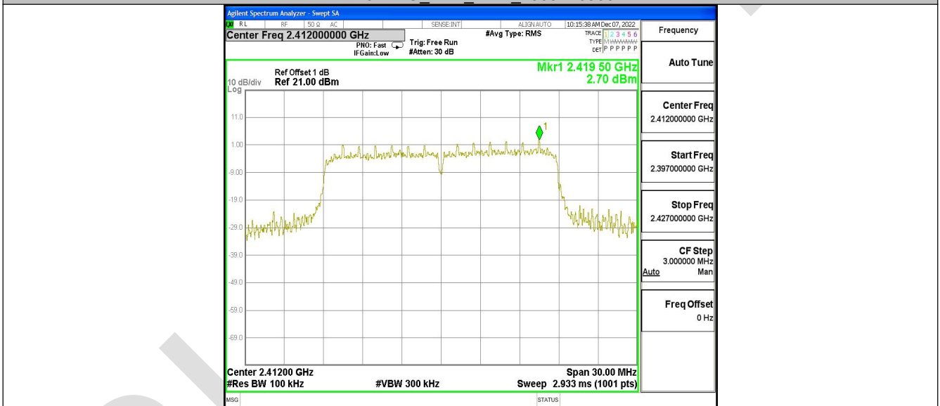
11N20MIMO_Ant2_2412_0~Reference
