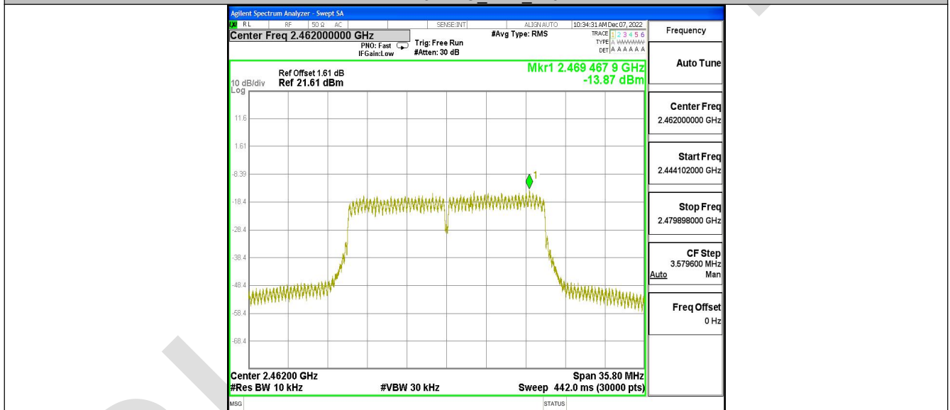
11N20MIMO_Ant2_2462
