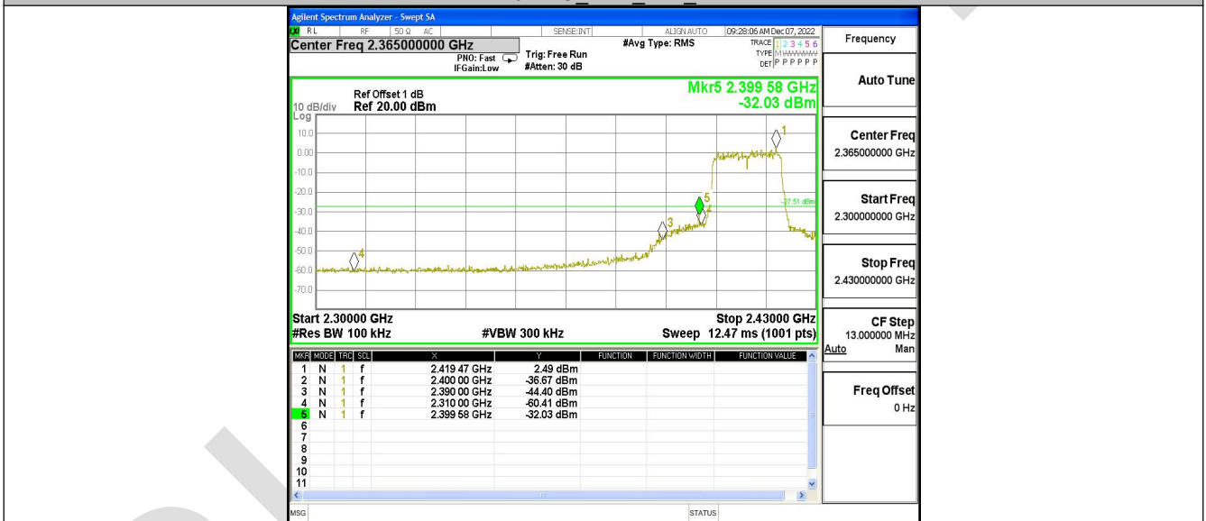
11N20SISO_Ant2_Low_2412
