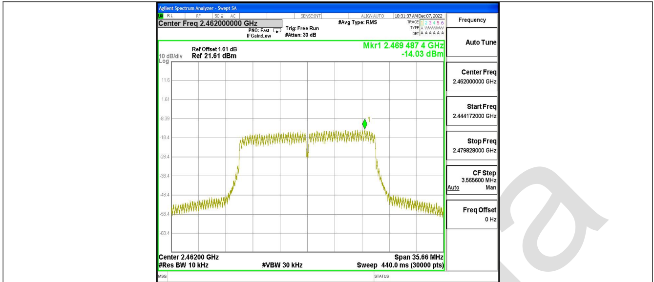
11N20MIMO_Ant1_2462
