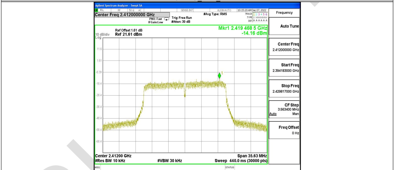
11N20MIMO_Ant2_2412
