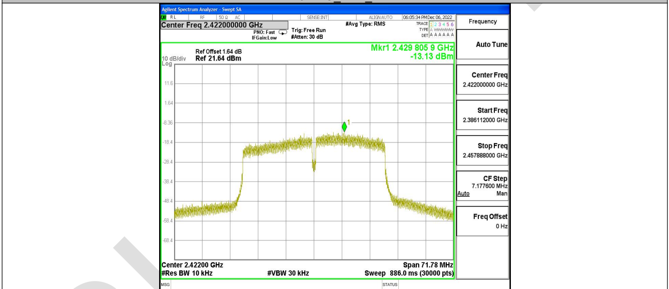
11N40SISO_Ant2_2422
