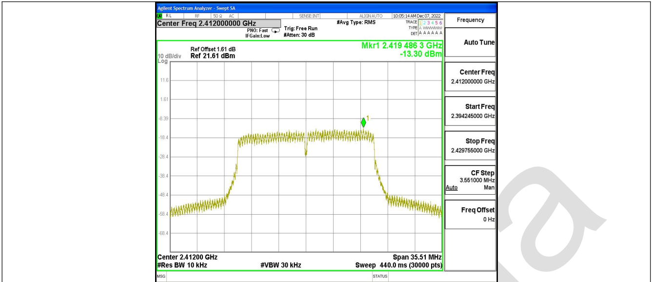
11N20MIMO_Ant1_2412
