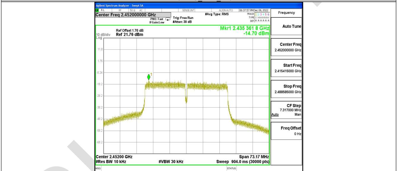
11N40SISO_Ant2_2452
