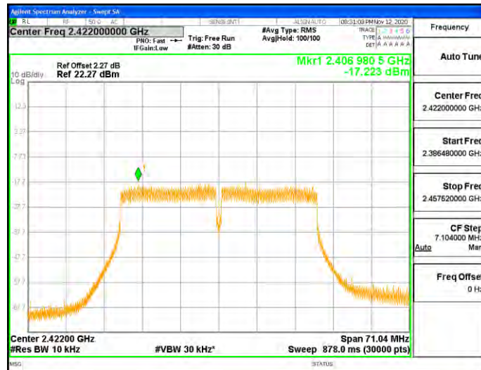
11N40SISO_Ant2_2422
