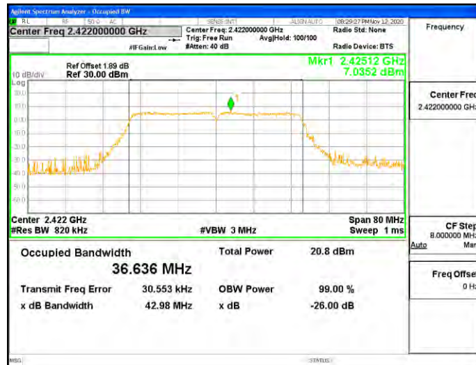
11N40_Ant2_2422
