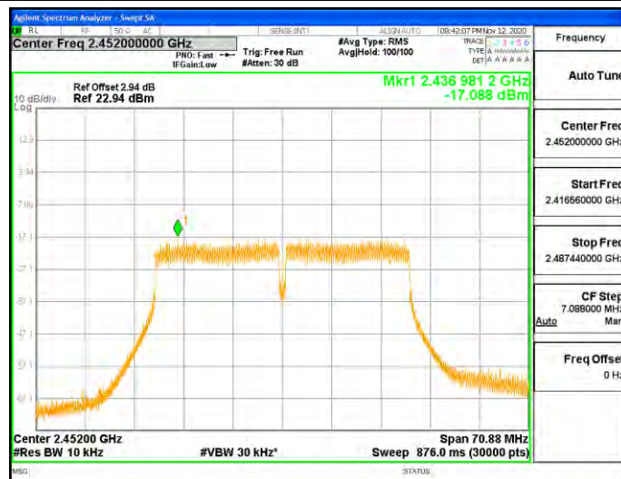
11N40SISO_Ant2_2452
