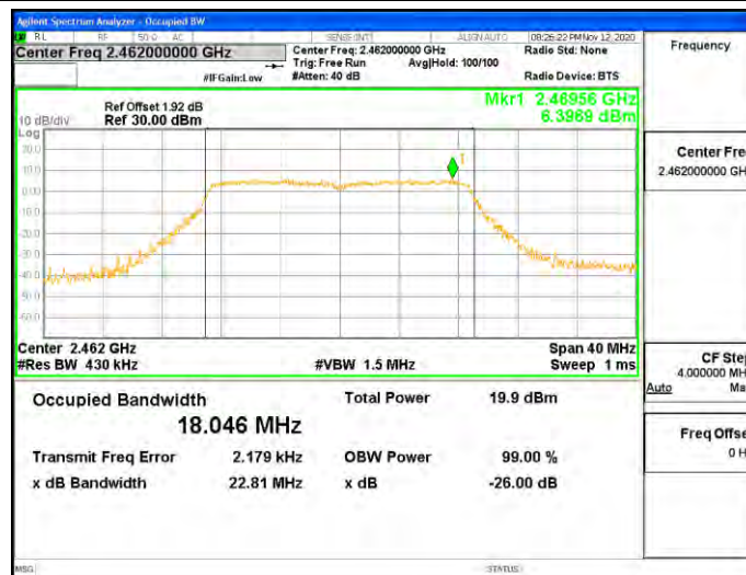
11N20_Ant2_2462
