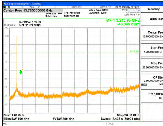
11N20SISO_Ant2_2412_0-Reference
