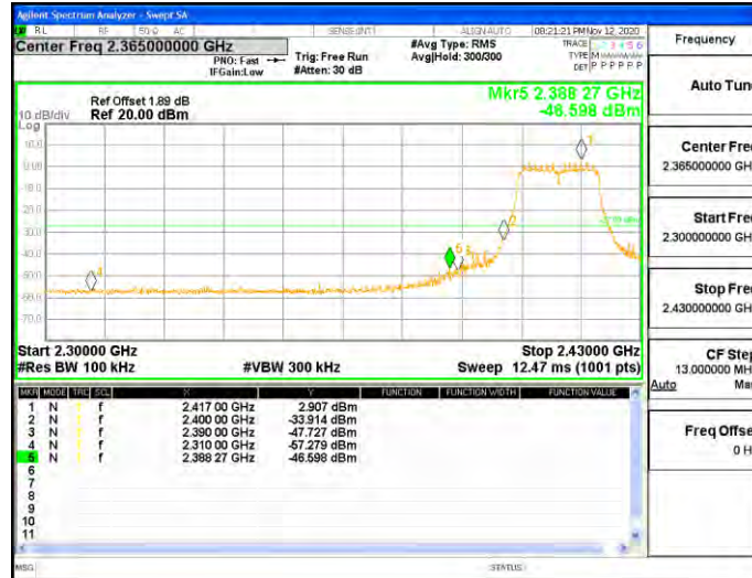
11N20SISO_Ant2_Low_2412
