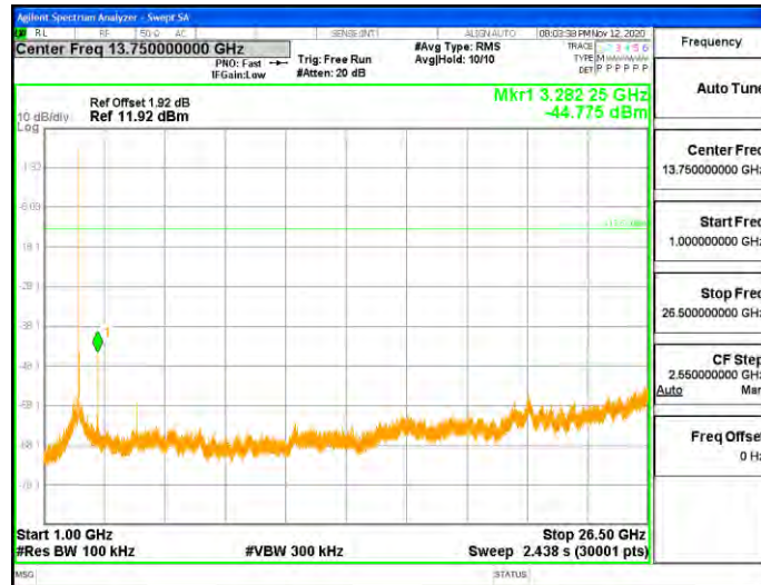
11B_Ant2_2462_0~Reference
