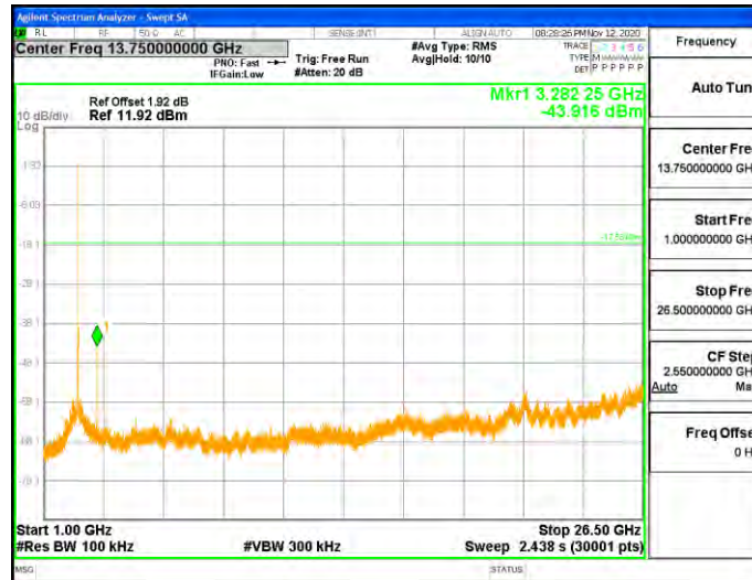
11N20SISO_Ant2_2462_0-Reference
