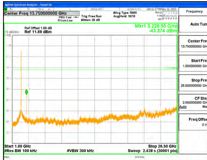
11N40SISO_Ant2_2422_0-Reference
