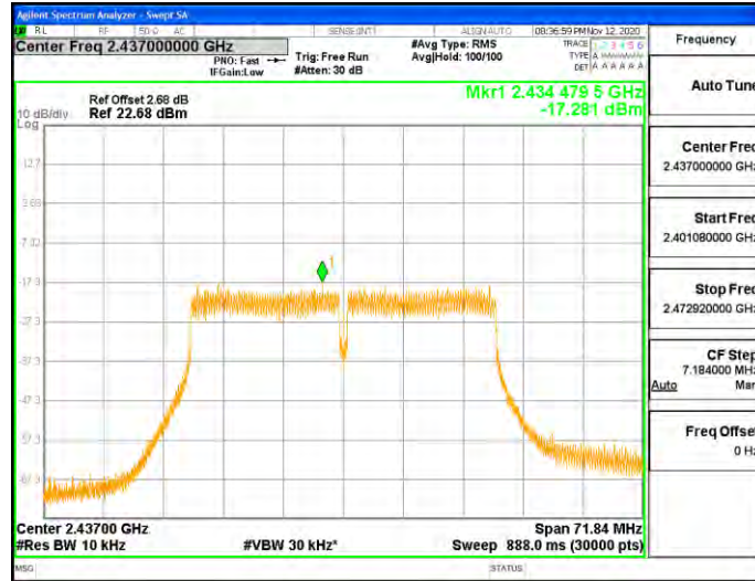
11N40SISO_Ant2_2437
