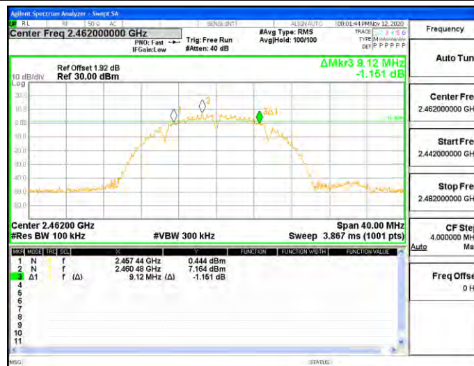
11B_Ant2_2462
