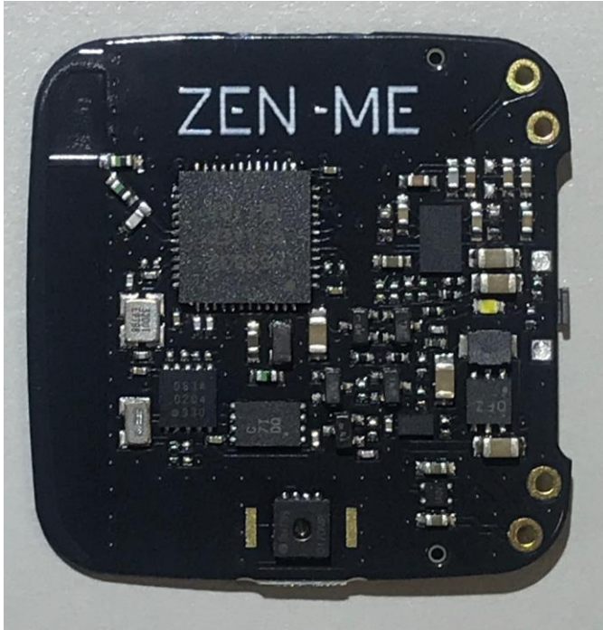
ZMH01A, ZMT01A PCB top
