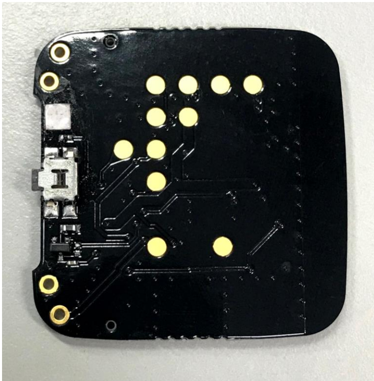
ZMH01A, ZMT01A PCB bottom
