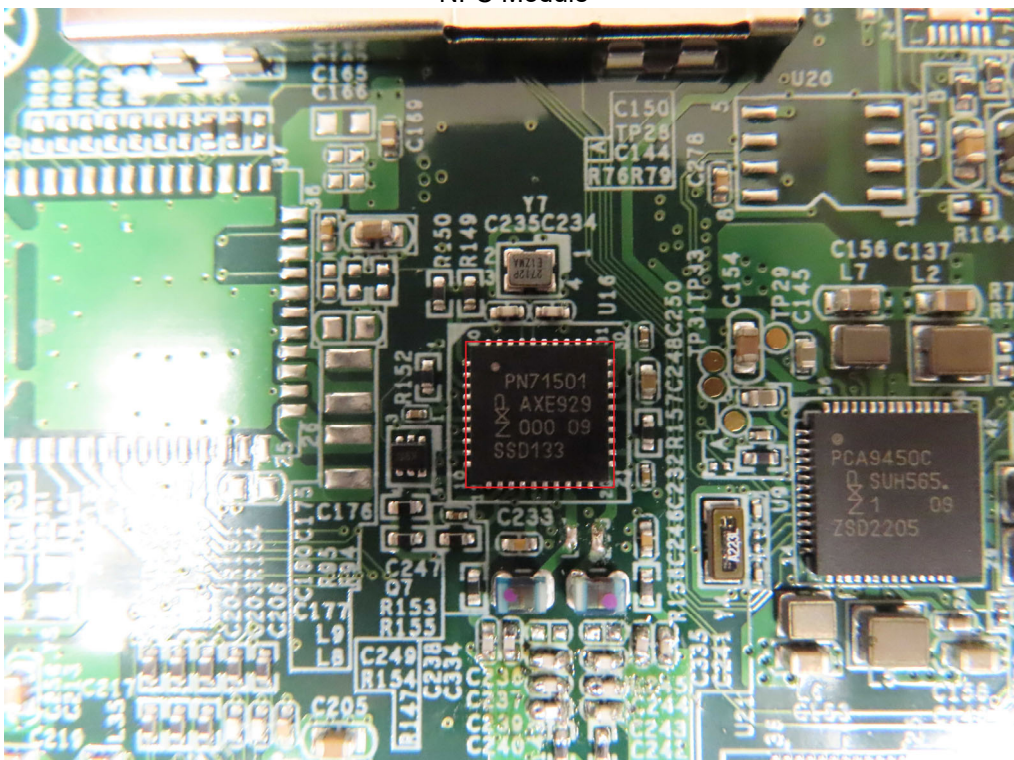
NFC Module
