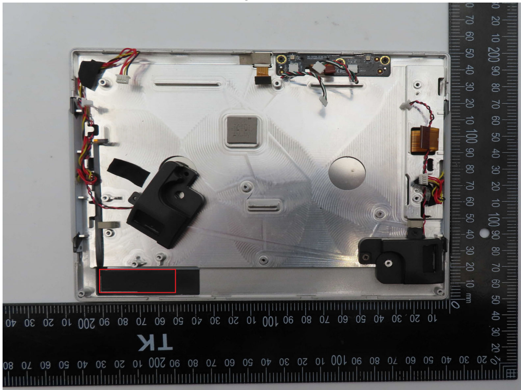
NFC Antenna
