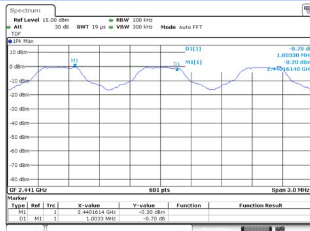
GFSK
