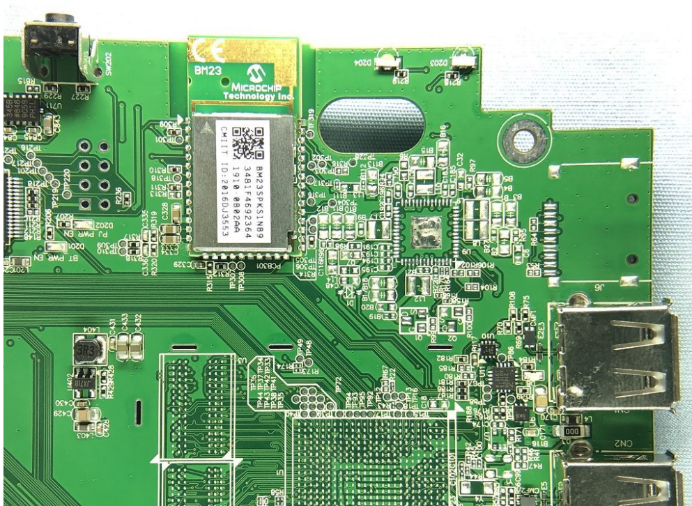
(10) EUT Photo
