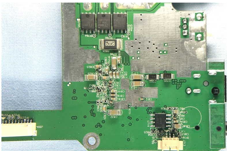
(6) EUT Photo
