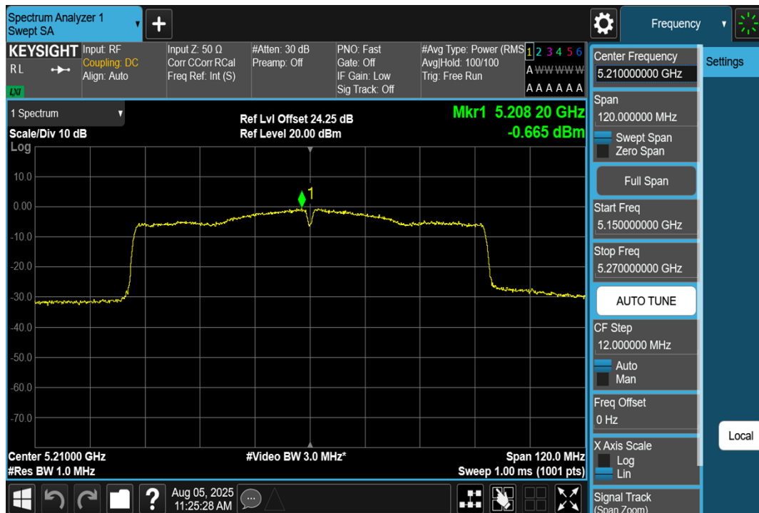
11AC80SISO-Ant1-5210-PASS
