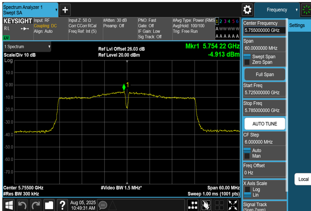
11N40SISO-Ant1-5755-PASS
