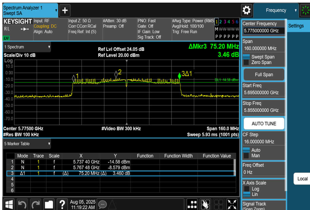
11AC80SISO-Ant1-5775-PASS
