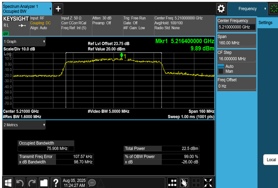
11AC80SISO-Ant1-5210
