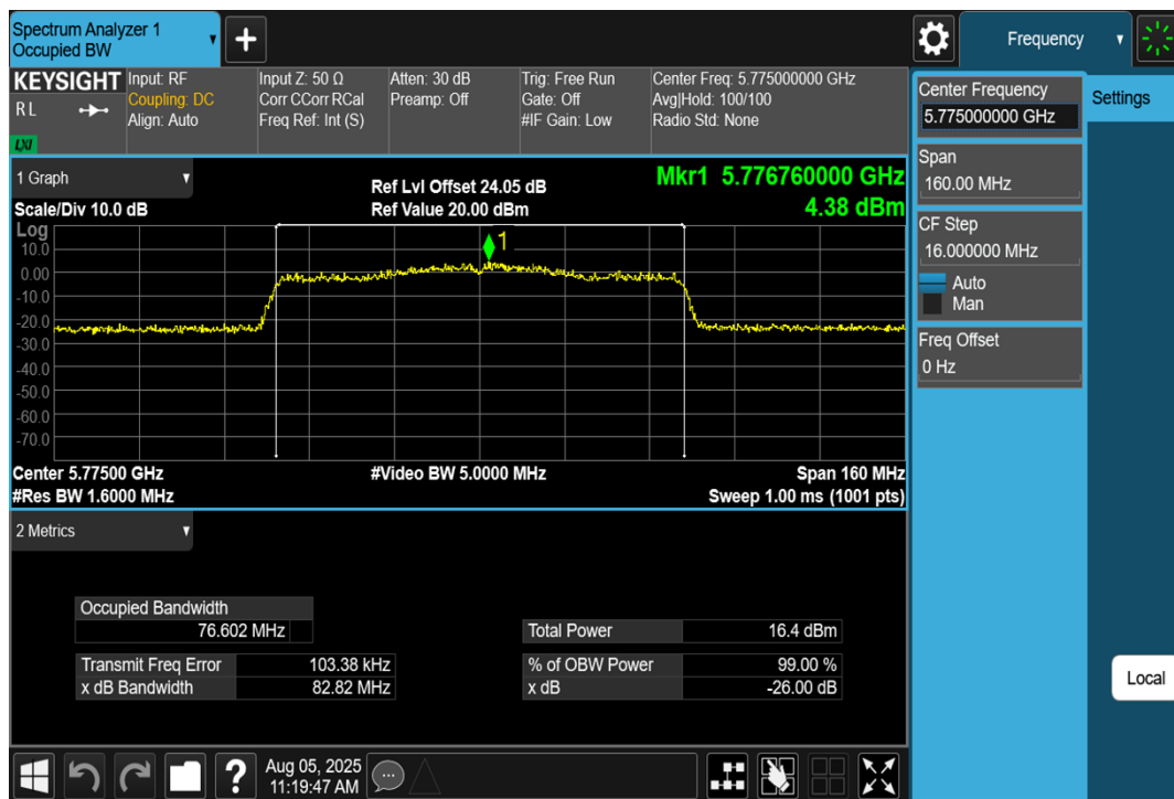
11AC80SISO-Ant1-5775
