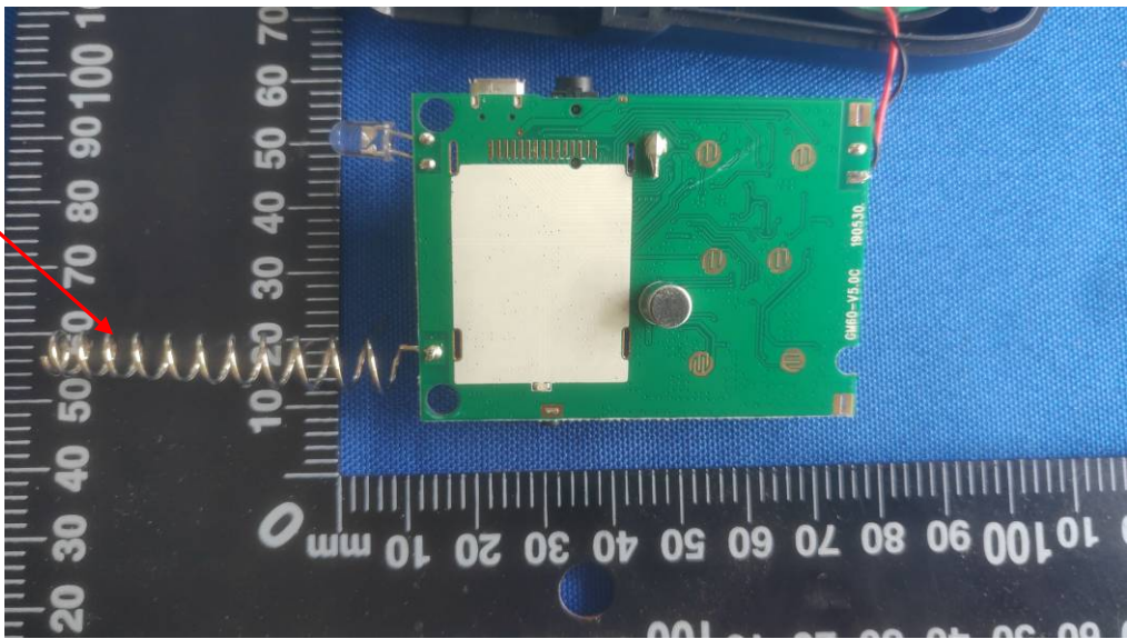
Antenna
