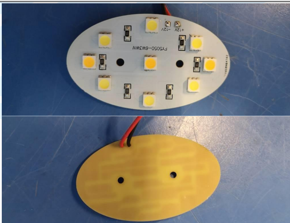
EUT Photo
