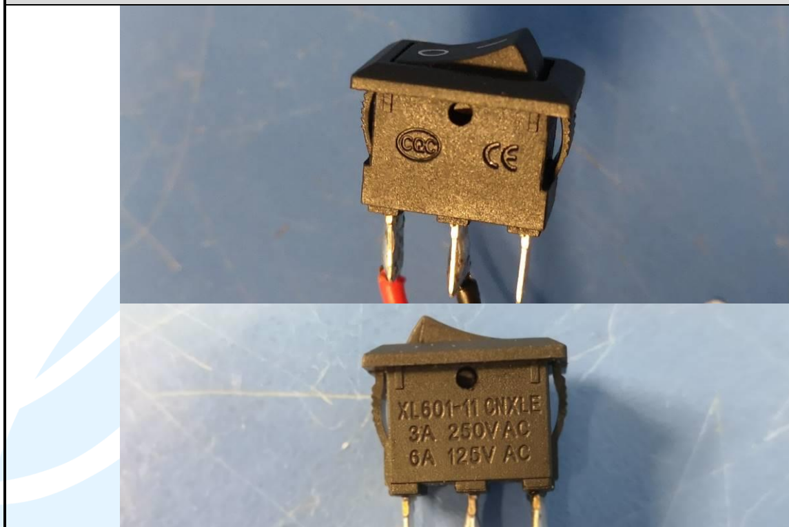
EUT Photo
