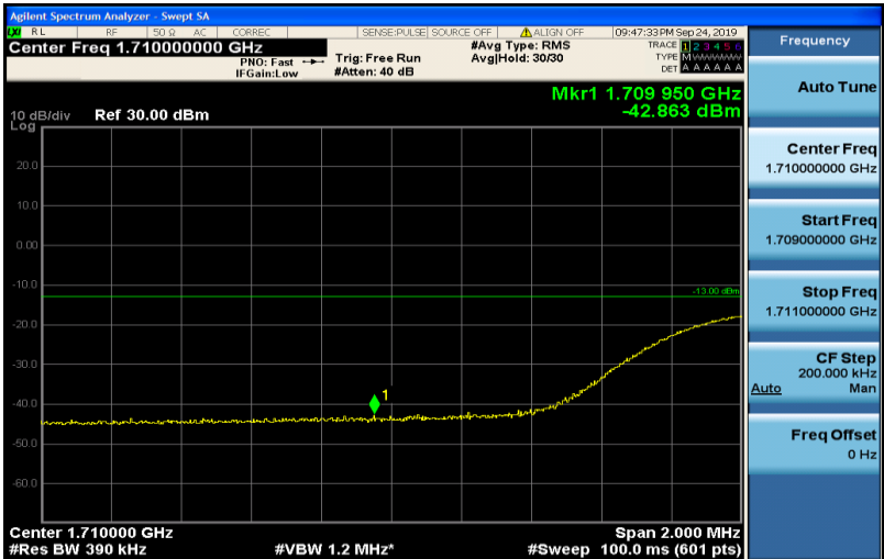
Band4-20MHz-QPSK-20050-100RB#0
