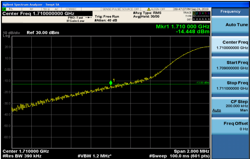
Band4-20MHz-QPSK-20050-1RB#99
