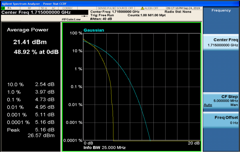
Band4-10MHz-QPSK-20000-50RB#0
