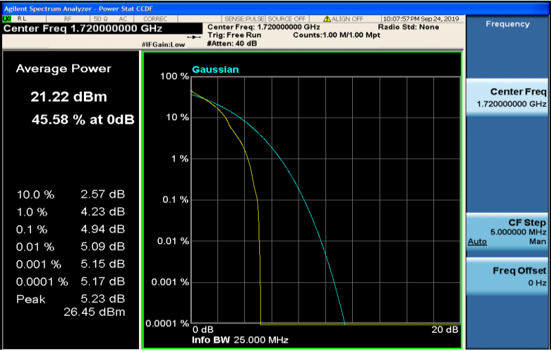
Band4-20MHz-QPSK-20050-100RB#0
