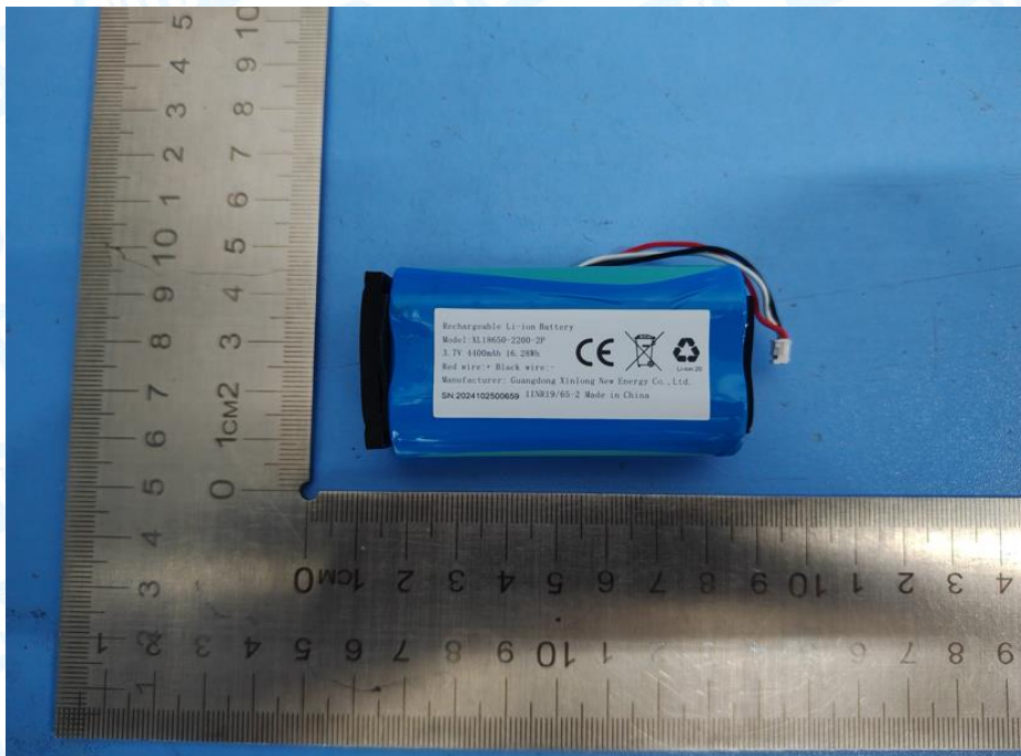
Photo 20 Battery parameters
