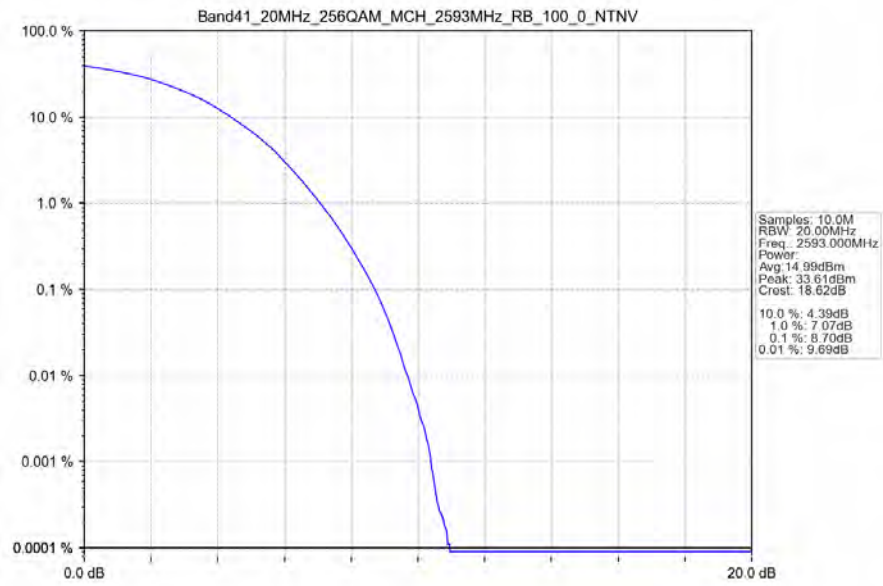
Band41_20MHz_256QAM_MCH_2593MHz_RB_100_0_NTNV
