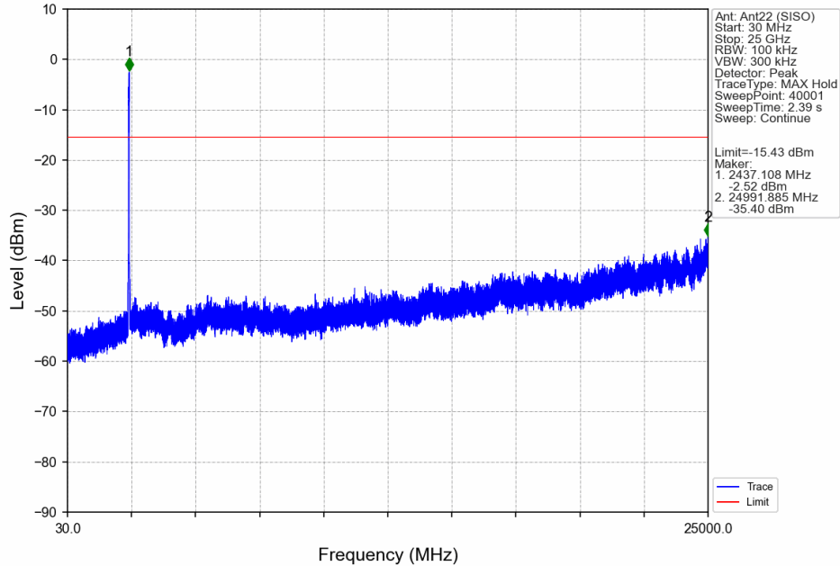
802.11n(HT40)_MCH_2437MHz_Ant22 (SISO)_NTNV
