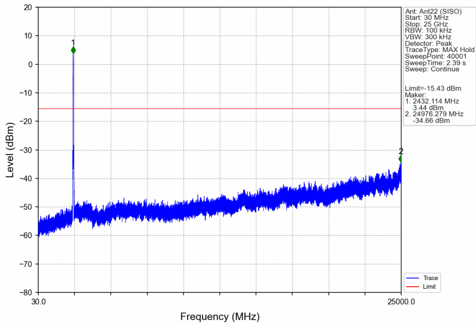
802.11n(HT40)_MCH_2437MHz_Ant22 (SISO)_NTNV
