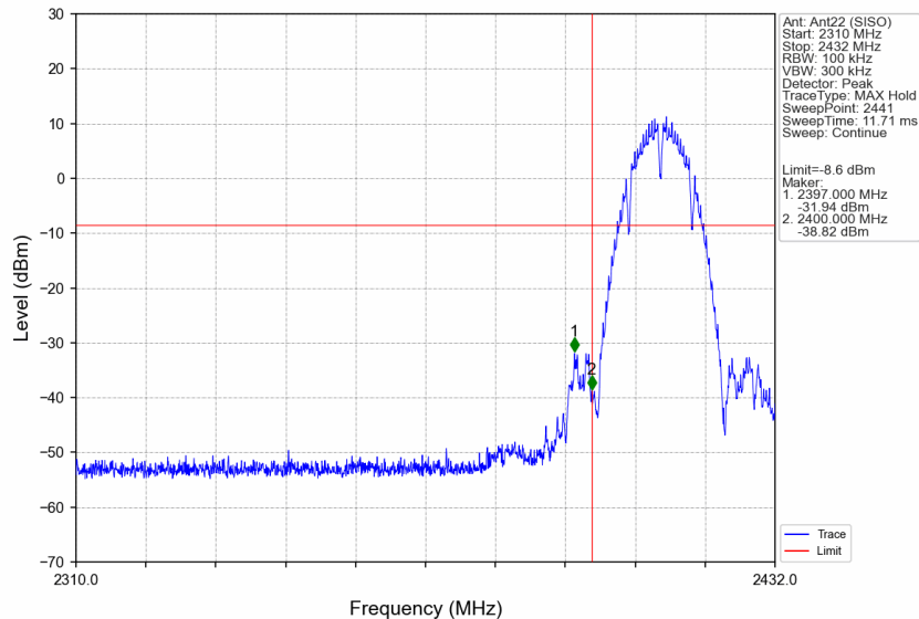
802.11b_LCH_2412MHz_Ant22 (SISO)_NTNV
