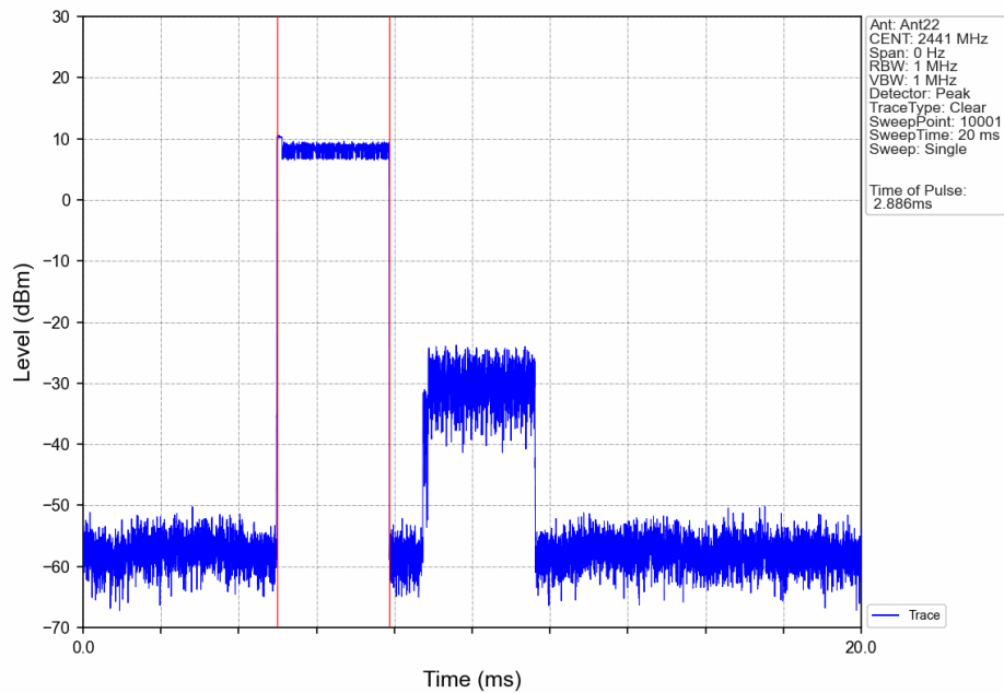
Pi/4DQPSK_2DH5_HOPP_Ant22_NTNV
