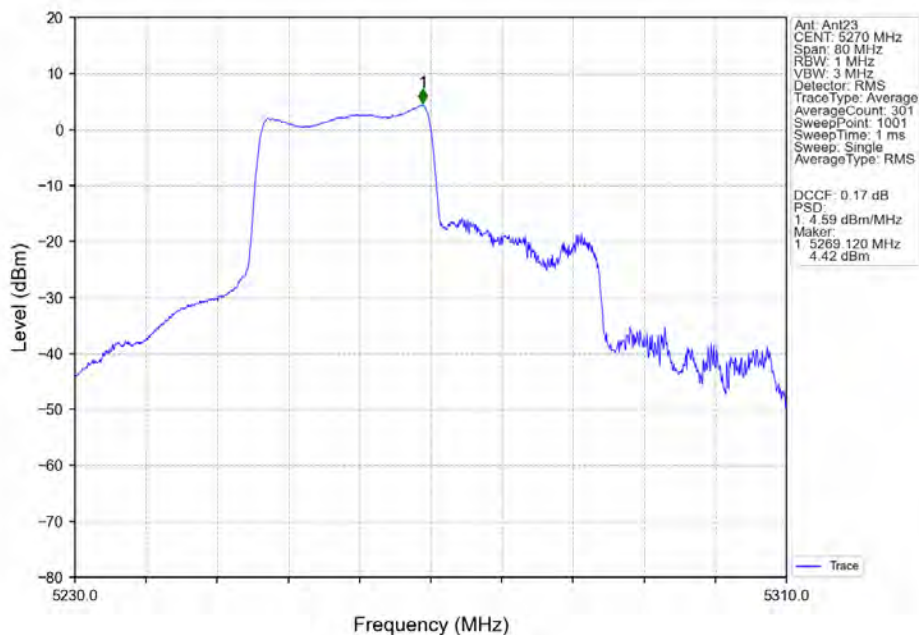
802.11ax(HEW40)_LCH_5270MHz_RU242_Left_Ant23_NTNV
