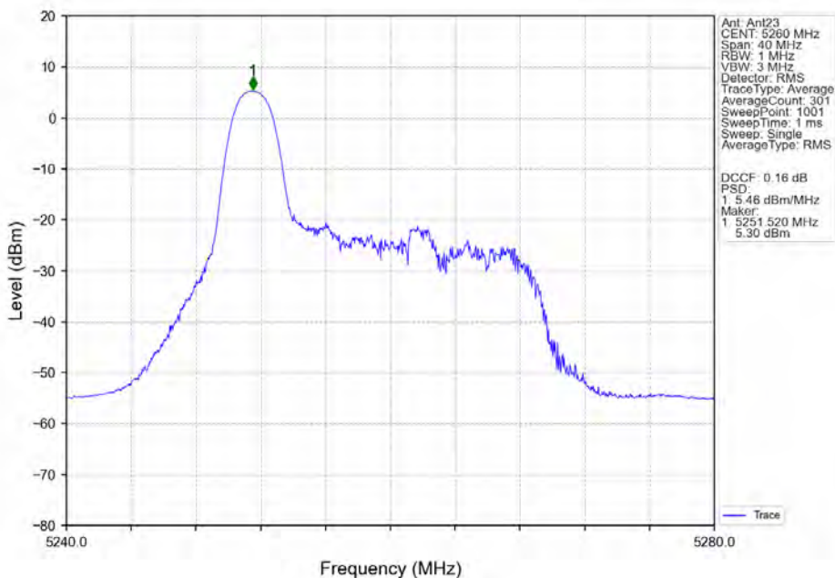
802.11ax(HEW20)_LCH_5260MHz_RU26_Left_Ant23_NTNV
