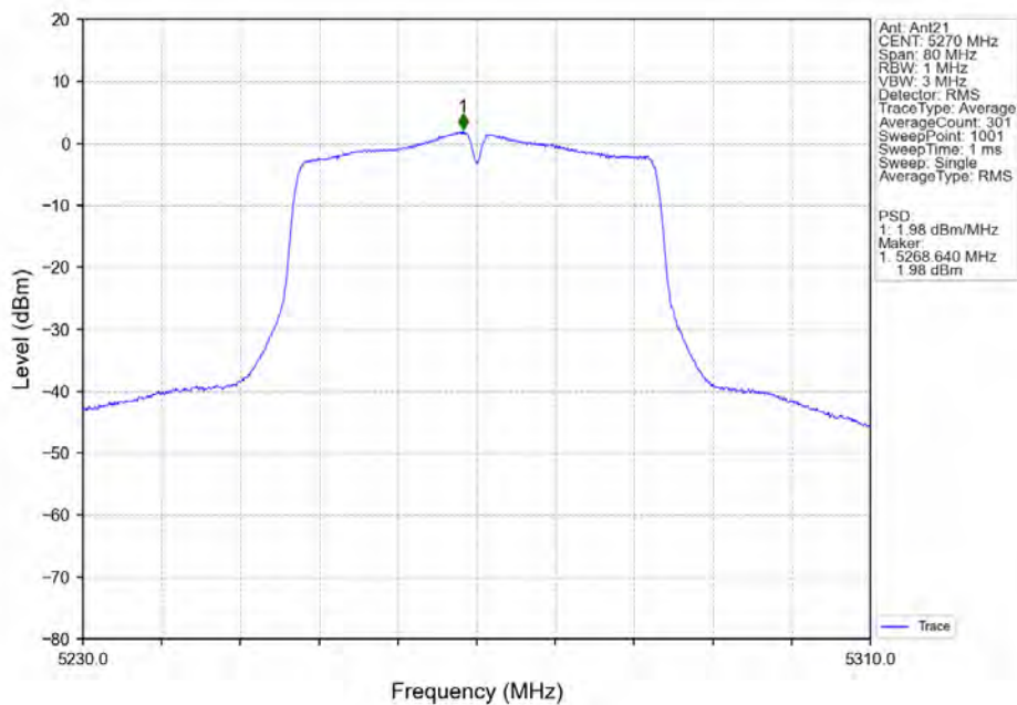
802.11n(HT40)_LCH_5270MHz_Ant21_NTNV
