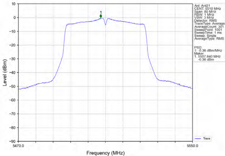
802.11n(HT40)_LCH_5510MHz_Ant21_NTNV
