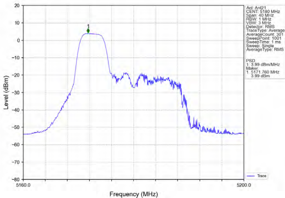
802.11ax(HEW20)_LCH_5180MHz_RU52_Left_Ant21_NTNV
