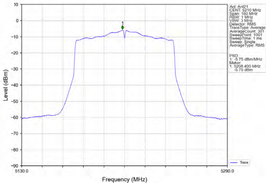
802.11ac(VHT80)_MCH_5210MHz_Ant21_NTNV
