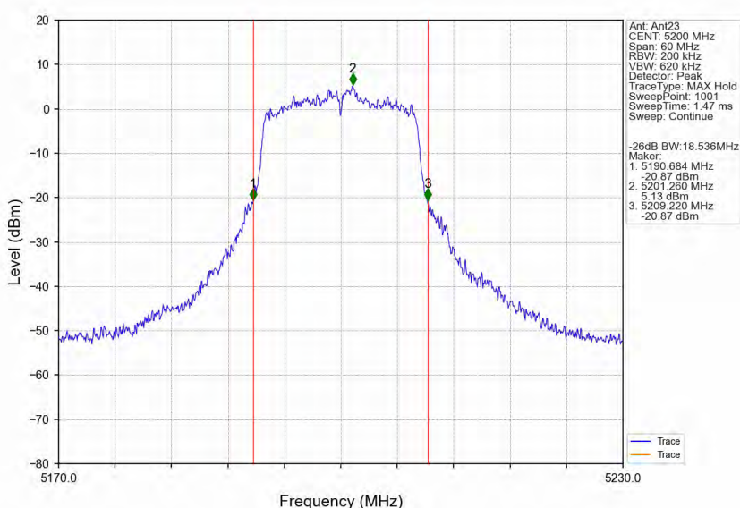
802.11a_MCH_5200MHz_Ant23_NTNV
