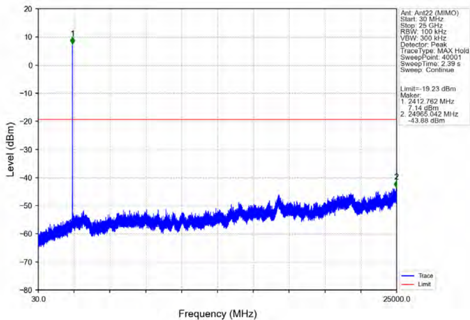
802.11b_LCH_2412MHz_Ant22 (MIMO)_NTNV
