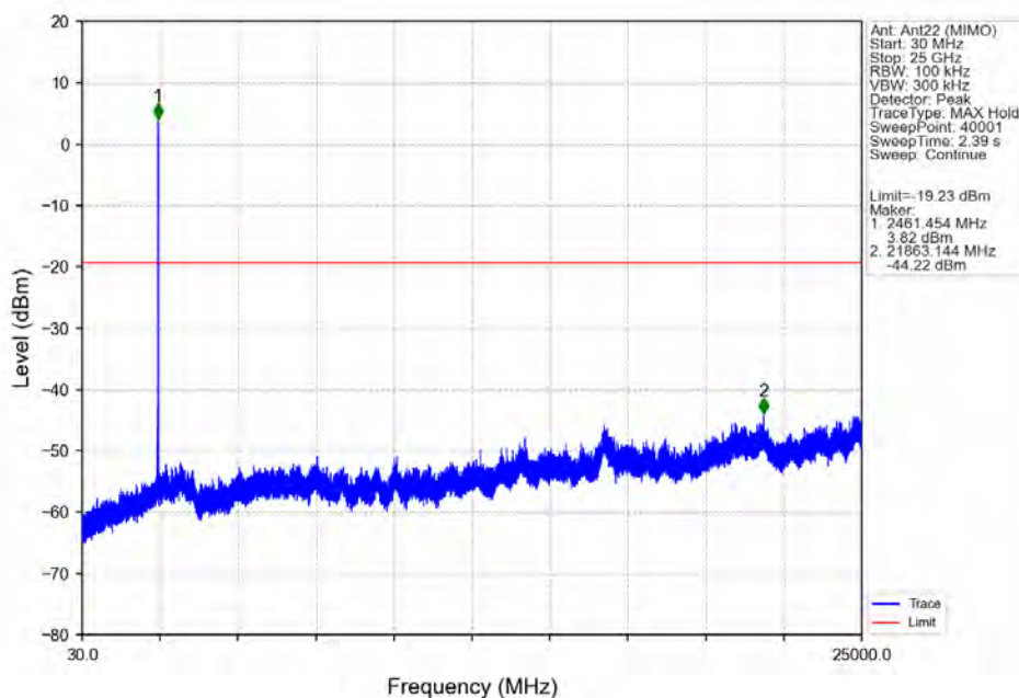
802.11b_HCH_2462MHz_Ant22 (MIMO)_NTNV
