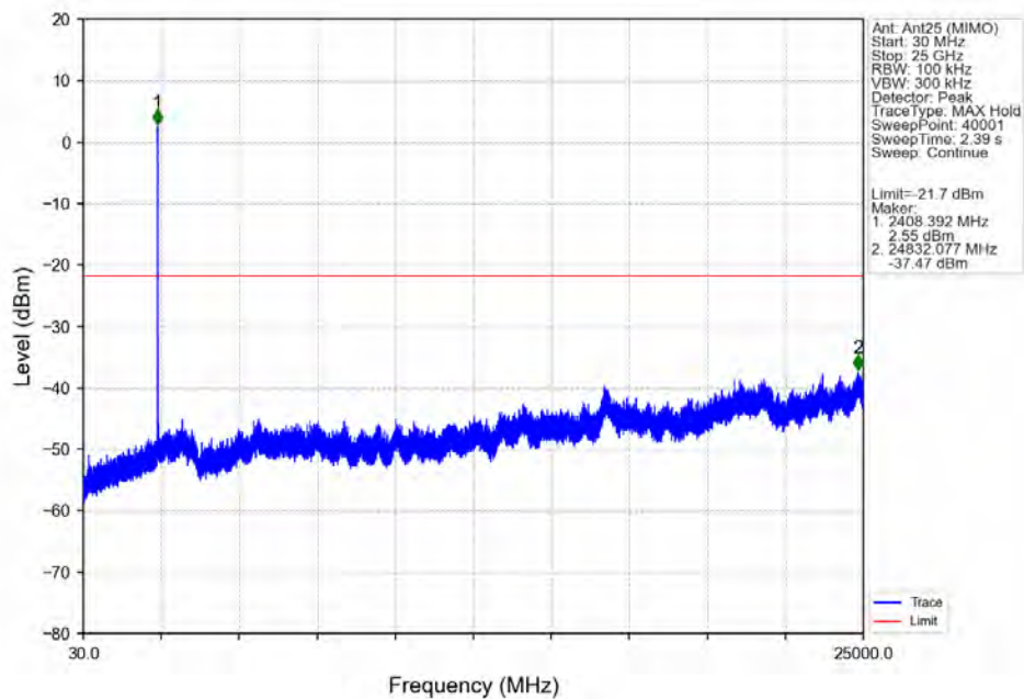
802.11g_LCH_2412MHz_Ant25 (MIMO)_NTNV
