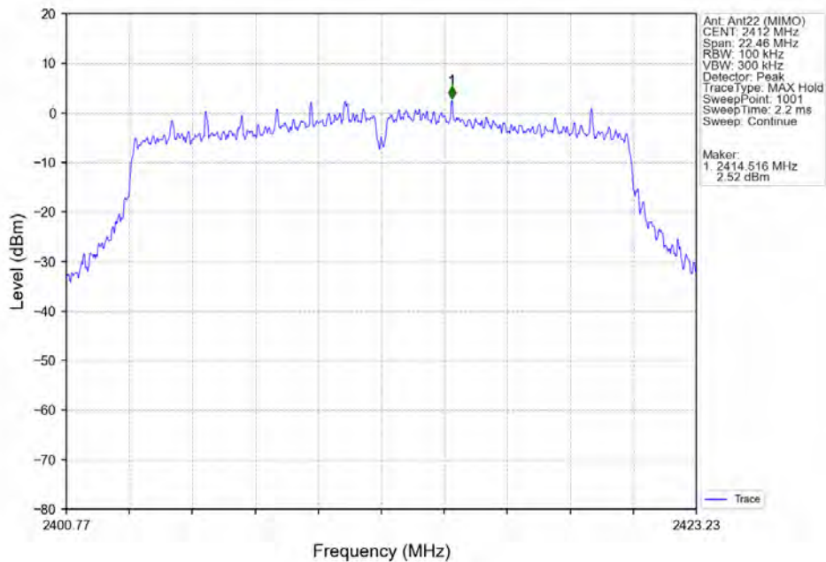
802.11n(HT20)_LCH_2412MHz_Ant22 (MIMO)_NTNV
