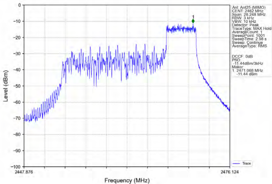
802.11ax(HEW20)_HCH_2462MHz_RU52_Right_Ant25 (MIMO)_NTNV
