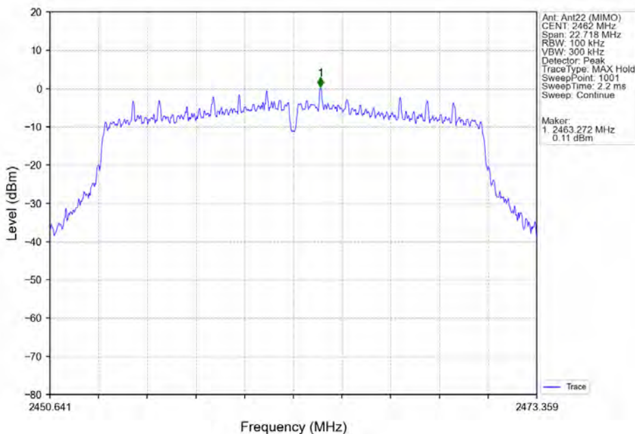
802.11n(HT20)_HCH_2462MHz_Ant22 (MIMO)_NTNV
