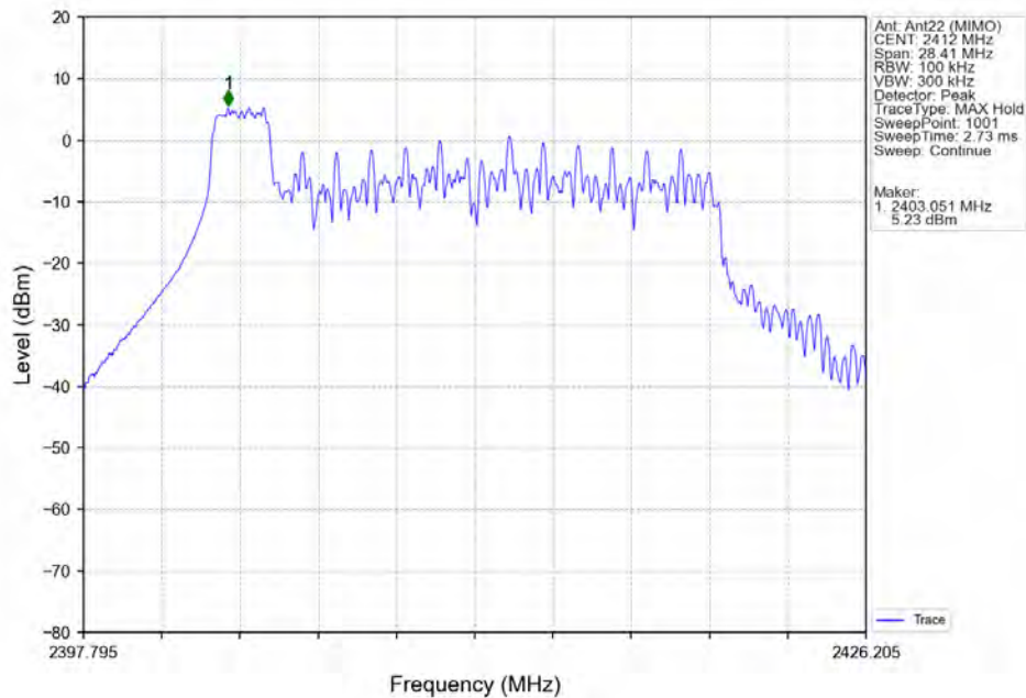
802.11ax(HEW20)_LCH_2412MHz_RU26_Left_Ant22 (MIMO)_NTNV
