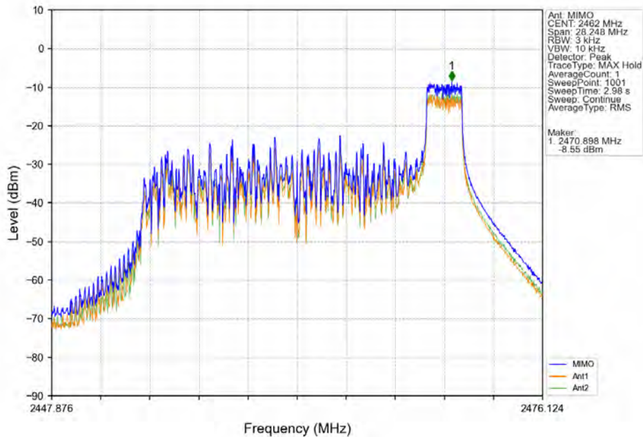
802.11ax(HEW20)_HCH_2462MHz_RU52_Right_Ant25 (MIMO)_NTNV
