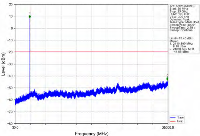
802.11b_LCH_2412MHz_Ant25 (MIMO)_NTNV
