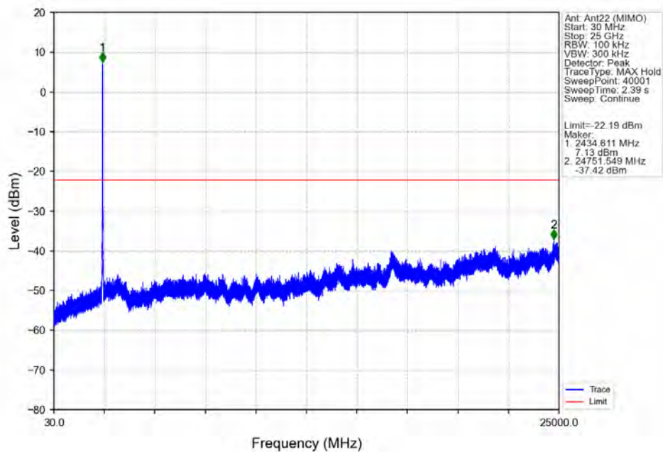
802.11g_MCH_2437MHz_Ant22 (MIMO)_NTNV
