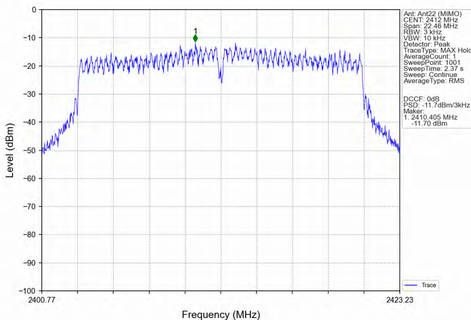
802.11n(HT20)_LCH_2412MHz_Ant22 (MIMO)_NTNV
