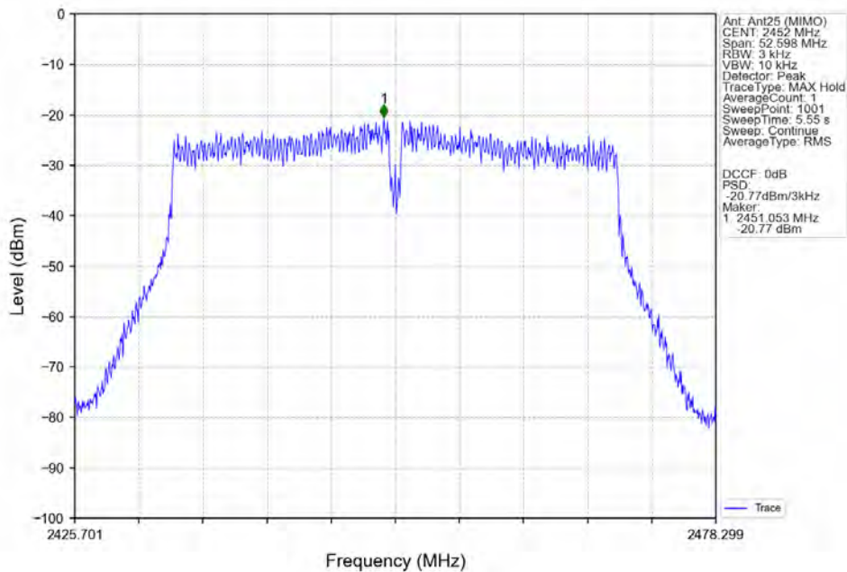
802.11n(HT40)_HCH_2452MHz_Ant25 (MIMO)_NTNV
