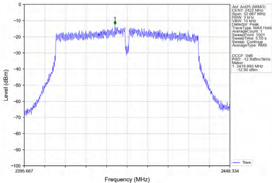
802.11n(HT40)_LCH_2422MHz_Ant25 (MIMO)_NTNV
