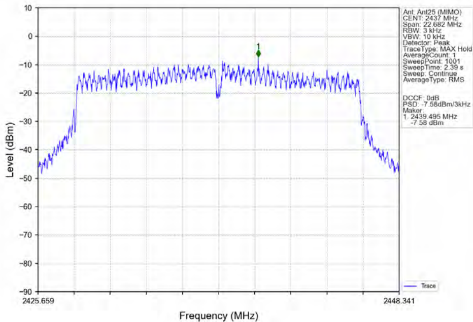
802.11n(HT20)_MCH_2437MHz_Ant25 (MIMO)_NTNV
