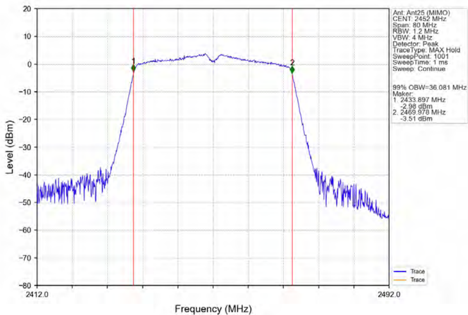
802.11n(HT40)_HCH_2452MHz_Ant25 (MIMO)_NTNV
