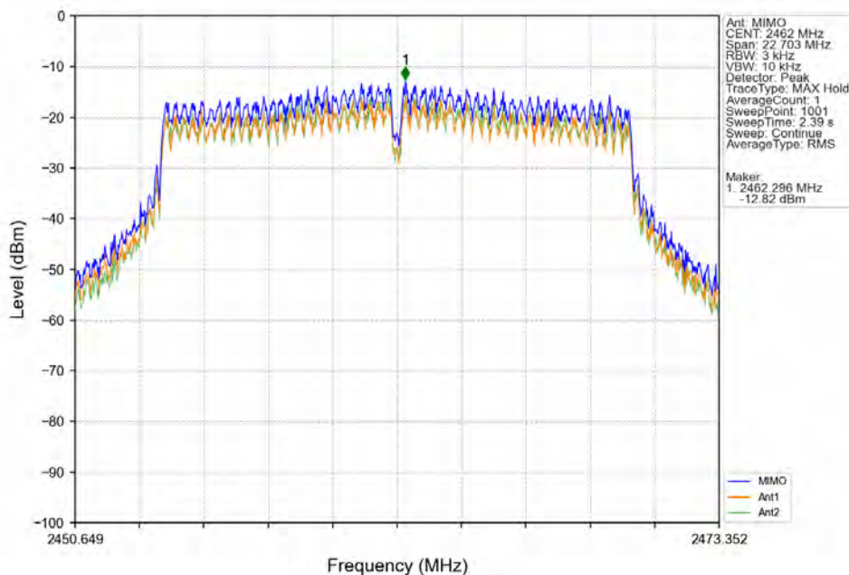
802.11g_HCH_2462MHz_MIMO_NTNV
