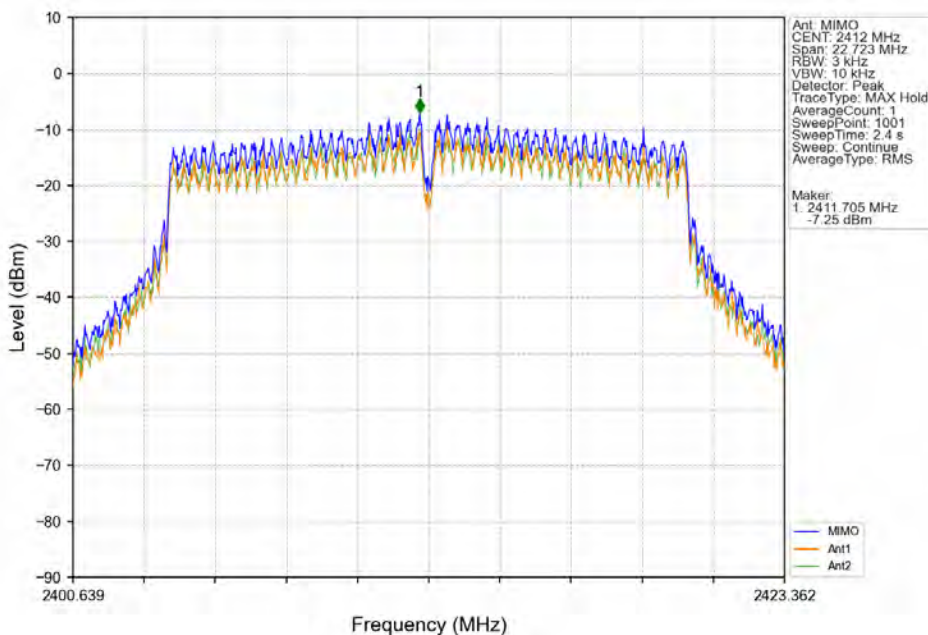
802.11g_LCH_2412MHz_MIMO_NTNV
