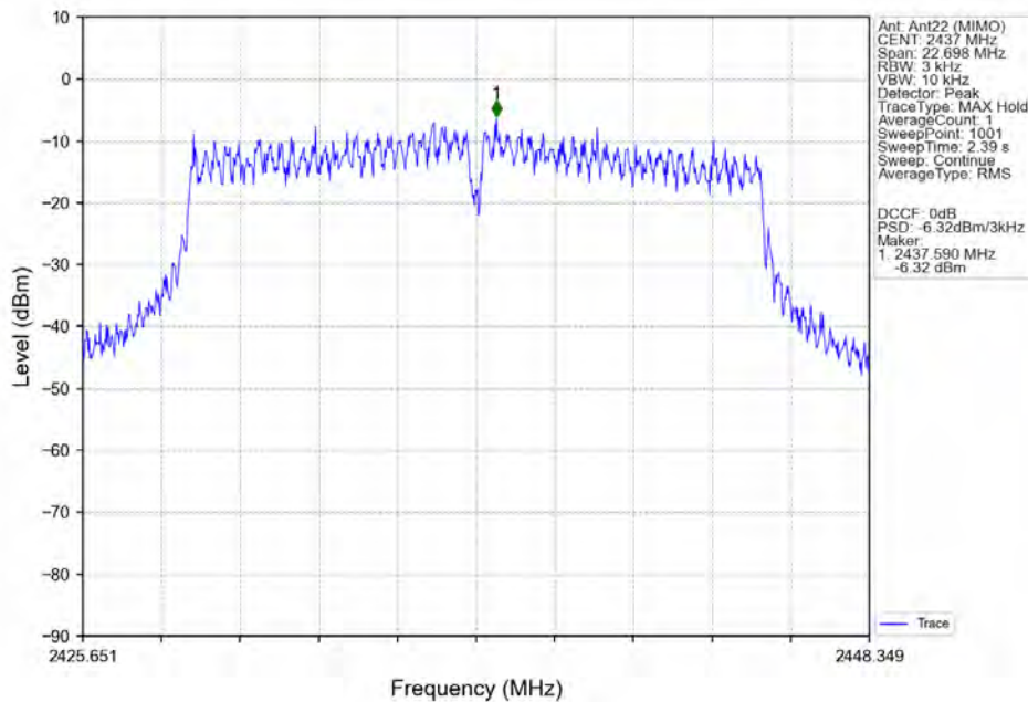
802.11g_MCH_2437MHz_Ant22 (MIMO)_NTNV
