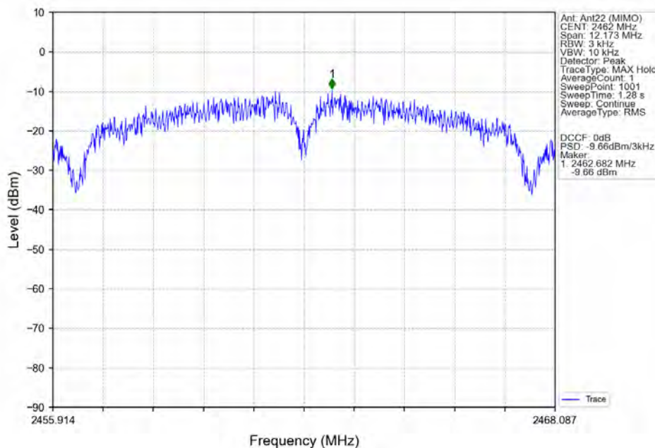
802.11b_HCH_2462MHz_Ant22 (MIMO)_NTNV
