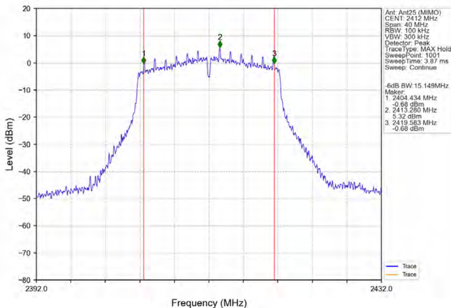
802.11g_LCH_2412MHz_Ant25 (MIMO)_NTNV
