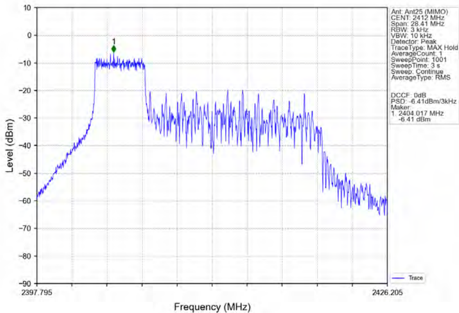
802.11ax(HEW20)_LCH_2412MHz_RU52_Left_Ant25 (MIMO)_NTNV
