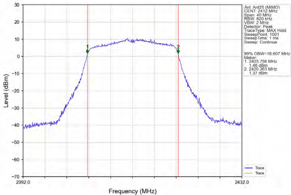
802.11g_LCH_2412MHz_Ant25 (MIMO)_NTNV
