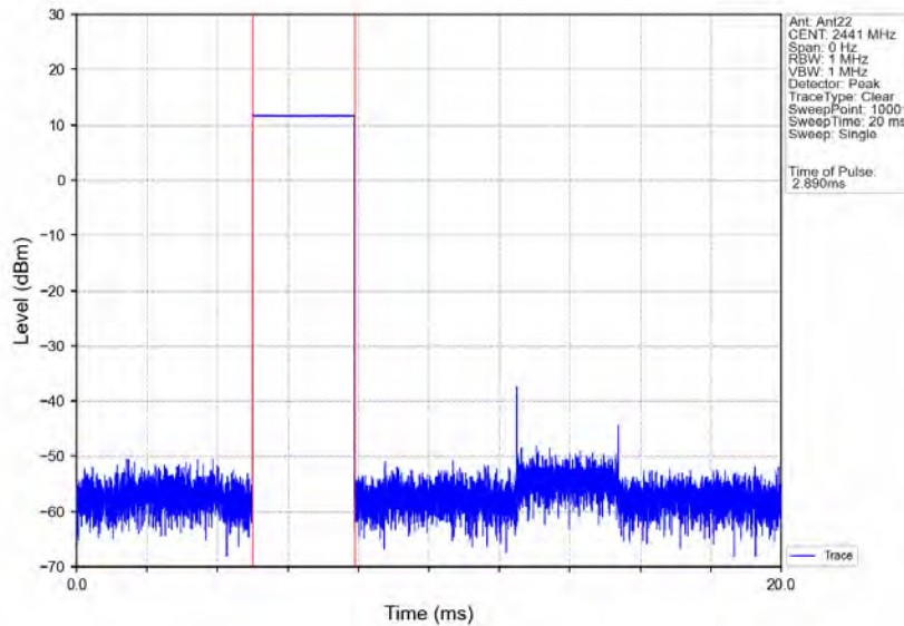
GFSK_DH5_HOPP_Ant22_NTNV
