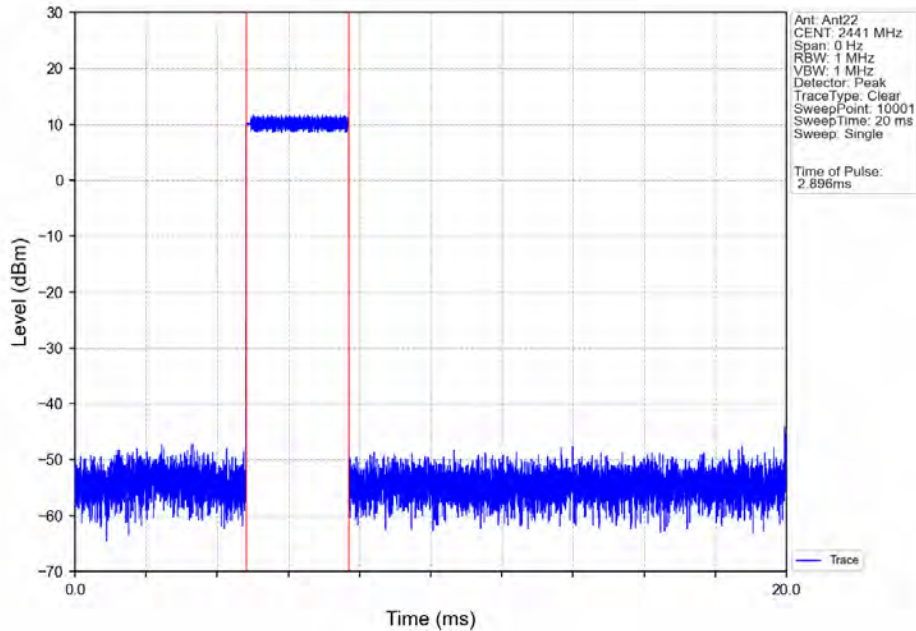
8DPSK_3DH5_HOPP_Ant22_NTNV
