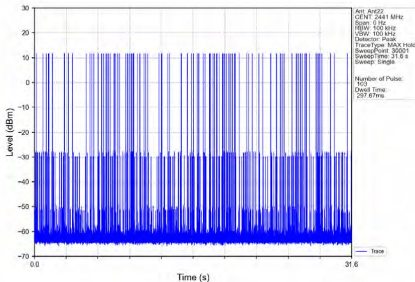
GFSK_DH5_HOPP_Ant22_NTNV
