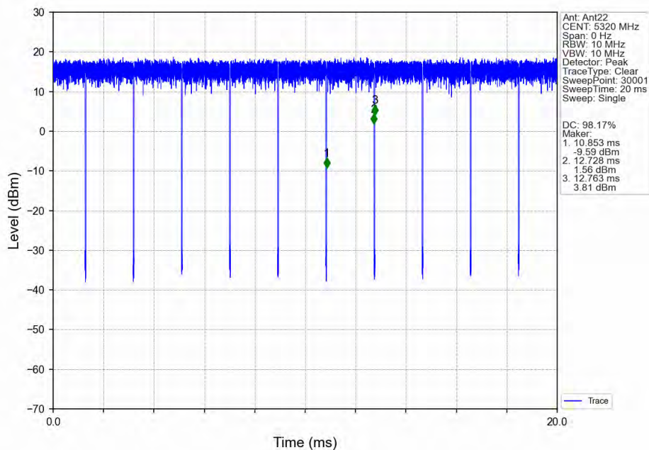
802.11n(HT20)_HCH_5320MHz_Ant22_NTNV
