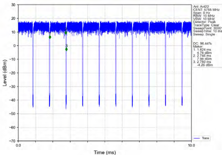
802.11n(HT40)_LCH_5755MHz_Ant22_NTNV
