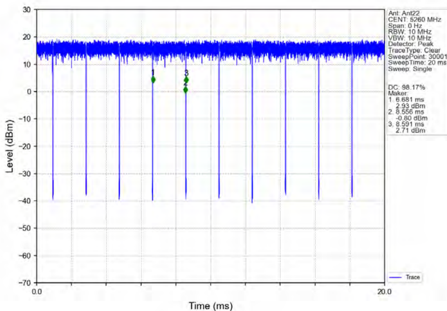
802.11n(HT20)_LCH_5260MHz_Ant22_NTNV
