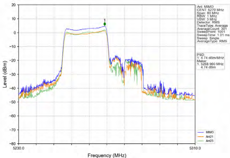
802.11ax(HE40) LCH_5270MHz_RU242_Left_MIMO_NTNV
