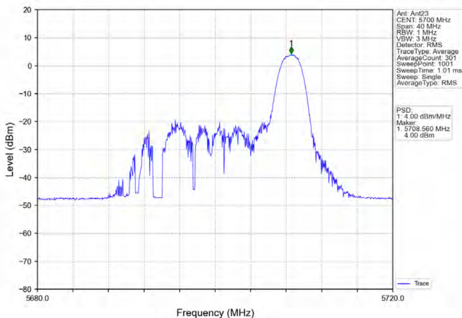
802.11ax(HE20) HCH_5700MHz_RU26_Right_Ant23_NTNV
