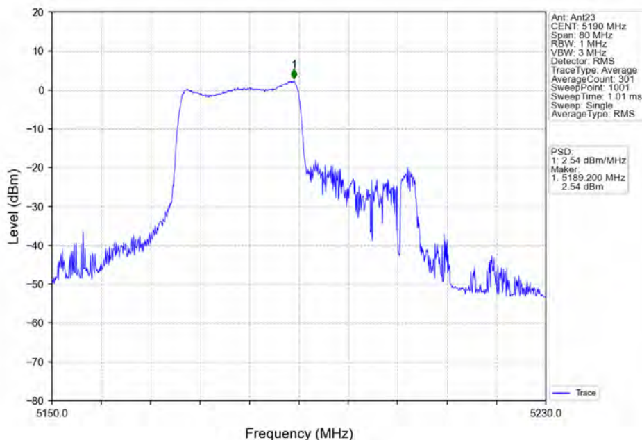
802.11ax(HE40) LCH_5190MHz RU242 Left MIMO_NTNV
