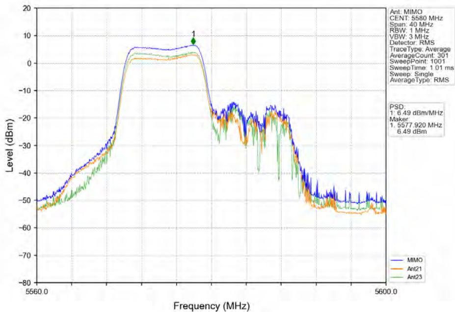
802.11ax(HE20) MCH 5580MHz RU106 Left MIMO NTNV
