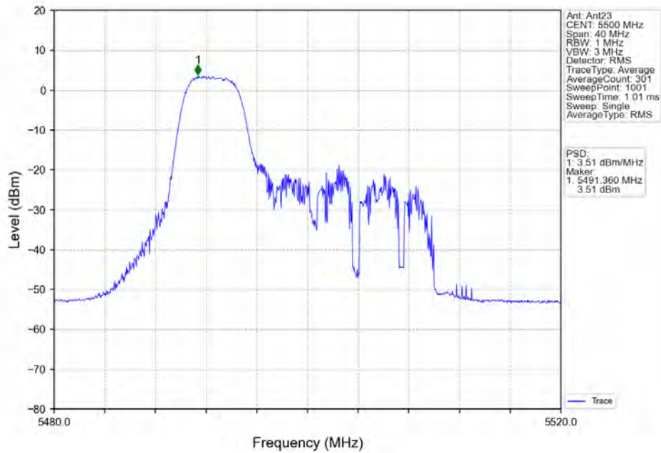
802.11ax(HE20) LCH 5500MHz RU52 Left MIMO NTN
