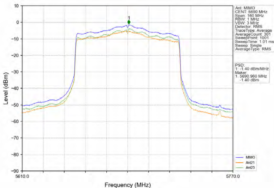
802.11ax(HE80) HCH 5690MHz RU996 Left MIMO NTNV
