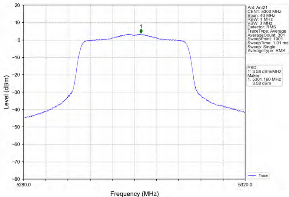
802.11ax(HE20) MCH 5300MHz RU242 Left Ant21 NTNV
