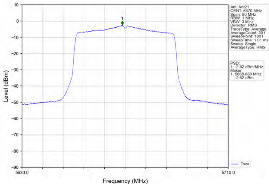
802.11ax(HE40) HCH 5670MHz RU484 Left Ant21 NTN
