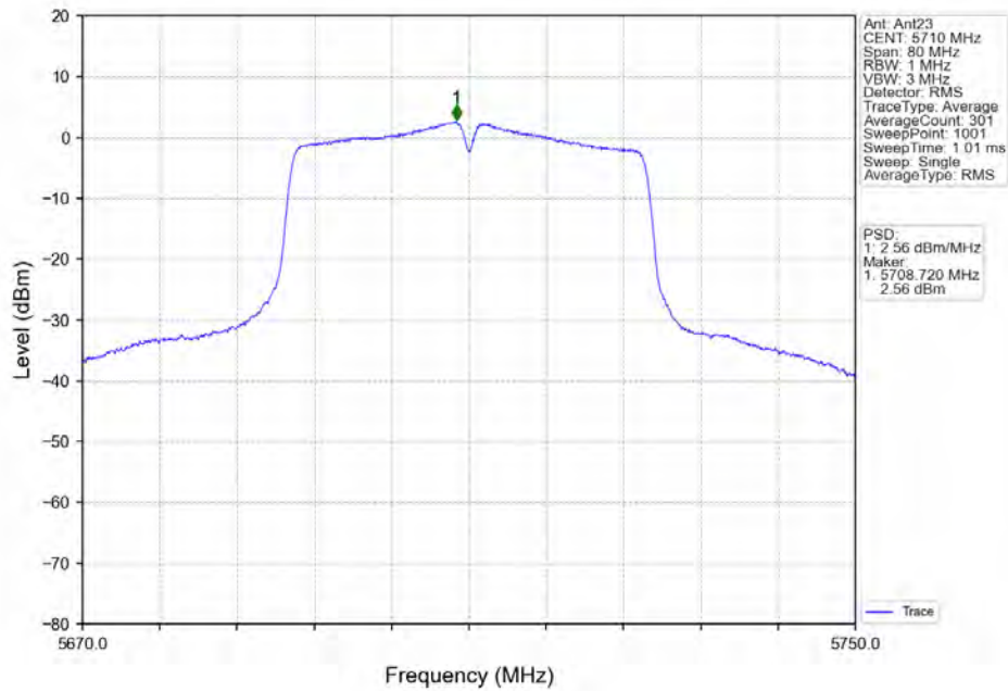
802.11ac(VHT40) HCH 5710MHz MIMO NTNV
