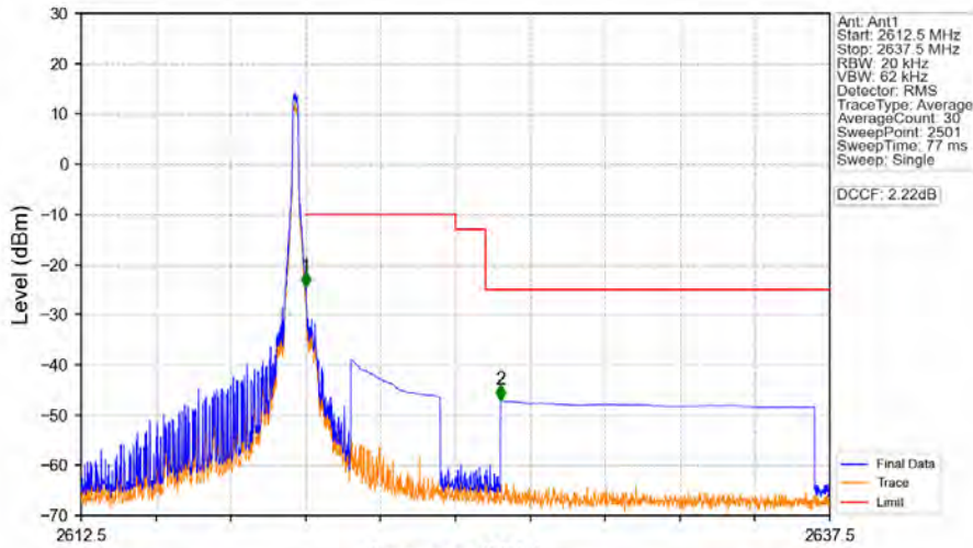
Band38_5MHz_QPSK_HCH_2617.5MHz_RB_1_24_NTNV
