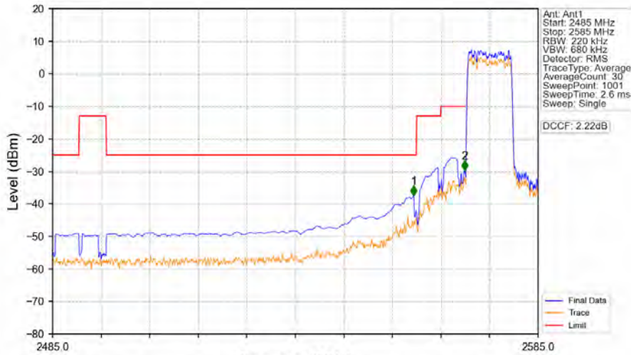
Band38_10MHz_QPSK_LCH_2575MHz_RB_50_0_NTNV
