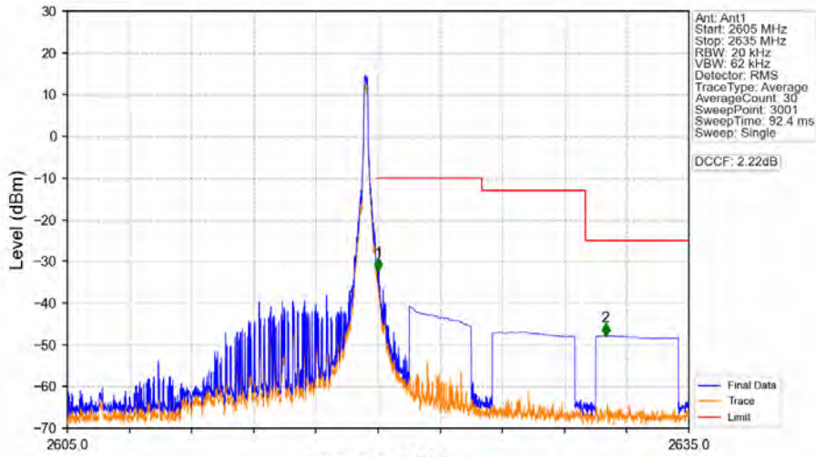
Band38_10MHz_QPSK_HCH_2615MHz_RB_1_49_NTNV
