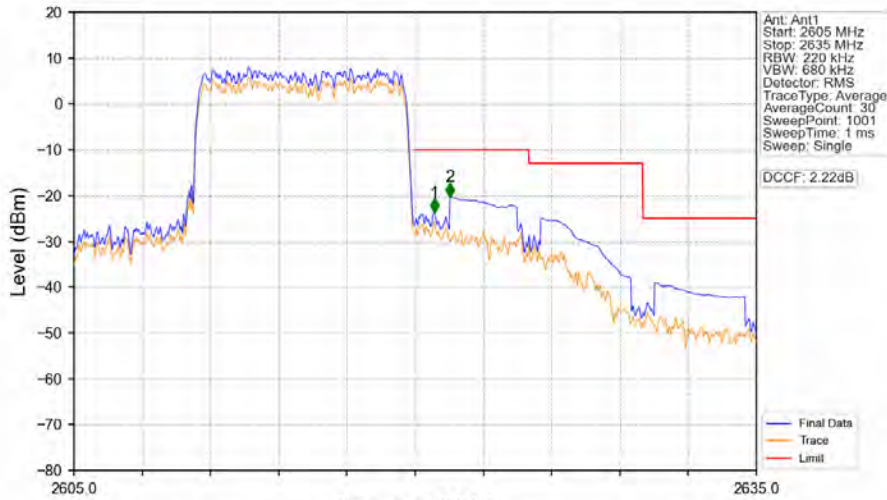
Band38_10MHz_QPSK_HCH_2615MHz_RB_50_0_NTNV
