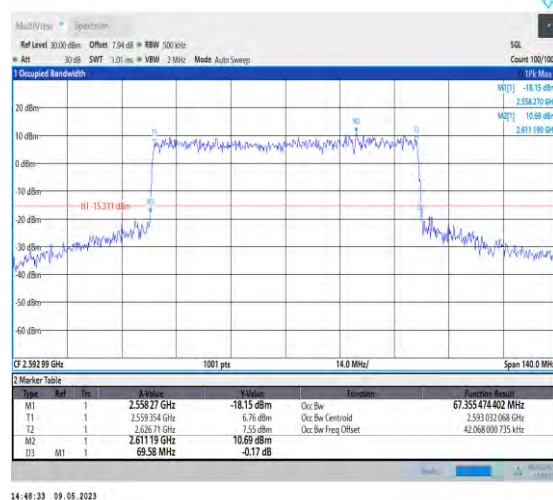
1-N41-PC3-30-70-M-6-CP-QPSK-Out_ Full-180@ 0-Ant1-67.355-69.580-≤70-PASS
