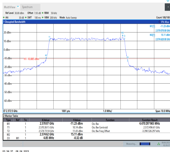
1-N38-PC3-15-5-L-1-DFT-QPSK-Outet_Full-25@0-A nt1-4.47-4.850-≤5-PASS
