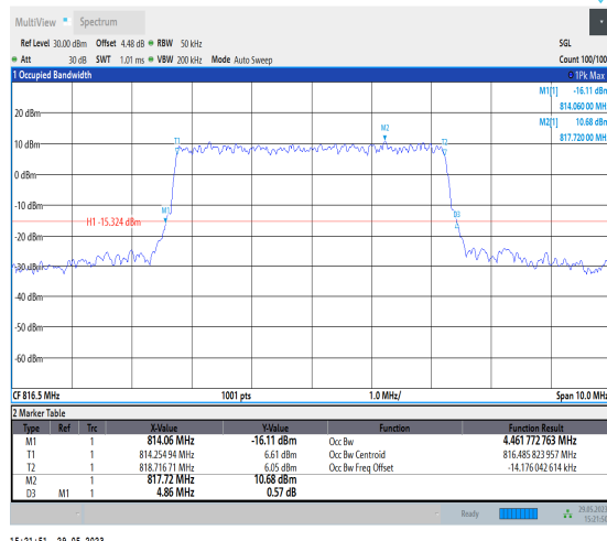
NTNV_N26-814-824_PC3_15_5_L_TID7_Ant1#1
