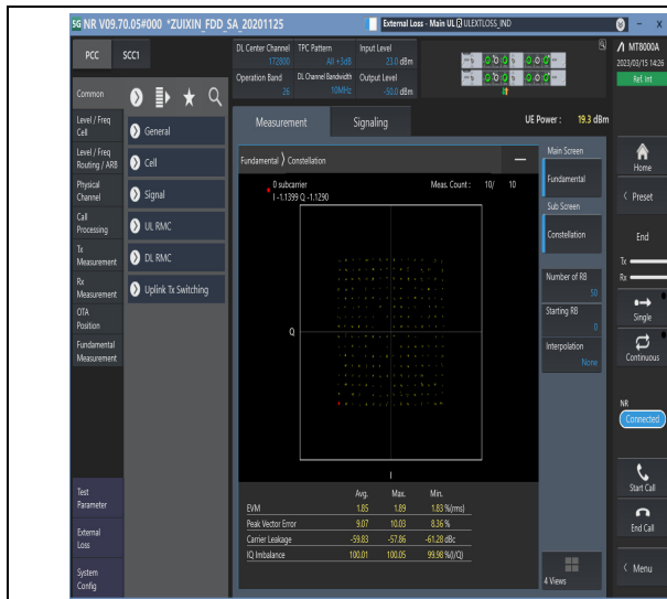
NTNV,N26-814-824,_PC3,_15,10,M,TID5,#1
