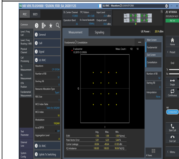
NTNV,N26-814-824,_PC3,_15,10,M,TID7,#1
