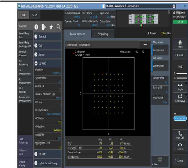
NTNV,N26-814-824,_PC3,_15,10,M,TID8,#1
