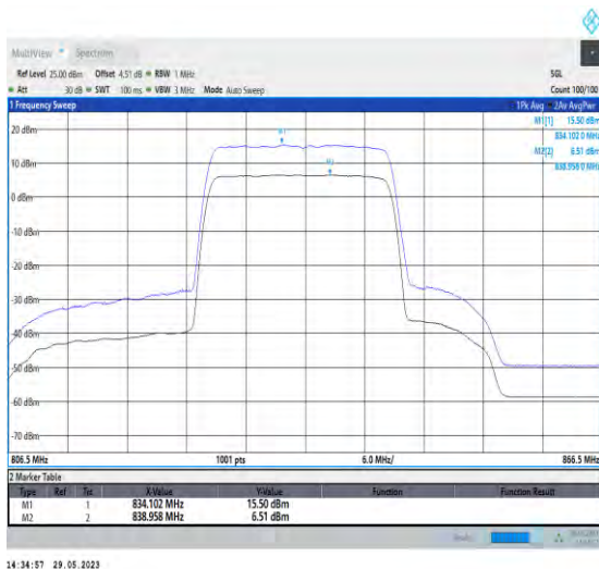
1-N5-PC3-15-20-M-1-DFT-256QAM-Outet_Full-100 @0-Ant1-8.99-100%-0.00-8.99-PASS-≤13
