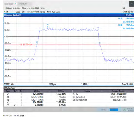
1-N5-PC3-15-5-L-2-DFT-P12BPSK-Outer_Full-25@0 -Ant1-4.478-4.830-≤5-PASS
