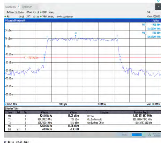
1-N5-PC3-15-5-L-4-DFT-64QAM-Outer_Full-25@0-A nt1-4.468-4.830-≤5-PASS
