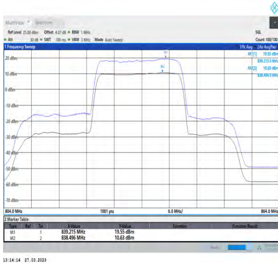
1-N5-PC3-15-20-L-1-DFT-256QAM-Outet_Full-100@ 0-Ant1-8.92-100%-0.00-8.92-PASS-≤13
