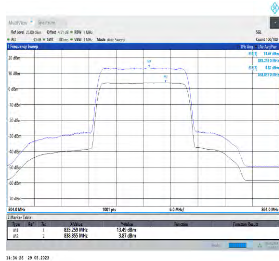
1-N5-PC3-15-20-L-2-CP-256QAM-Outet_Full-106@ 0-Ant1-9.62-100%-0.00-9.62-PASS-≤13
