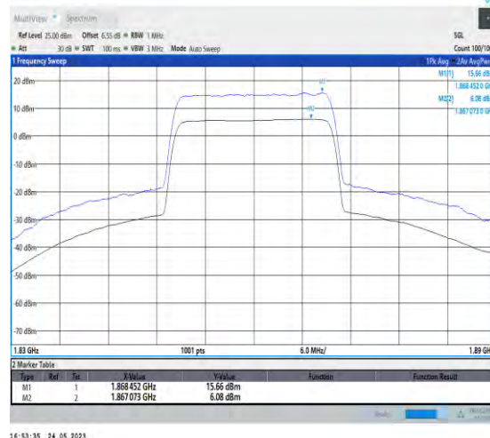
1-N2-PC3-15-20-L-2-CP-256QAM-Outter_Full-106@ 0-Ant1-9.58-100%-0.00-9.58-PASS-≤13
