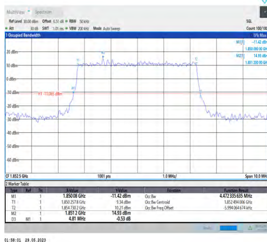
1-N2-PC3-15-5-L-2-DFT-P12BPSK-Outet_Full-25@0 -Ant1-4.472-4.810-≤5-PASS
