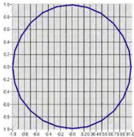
Isotropy @ 835MHz
