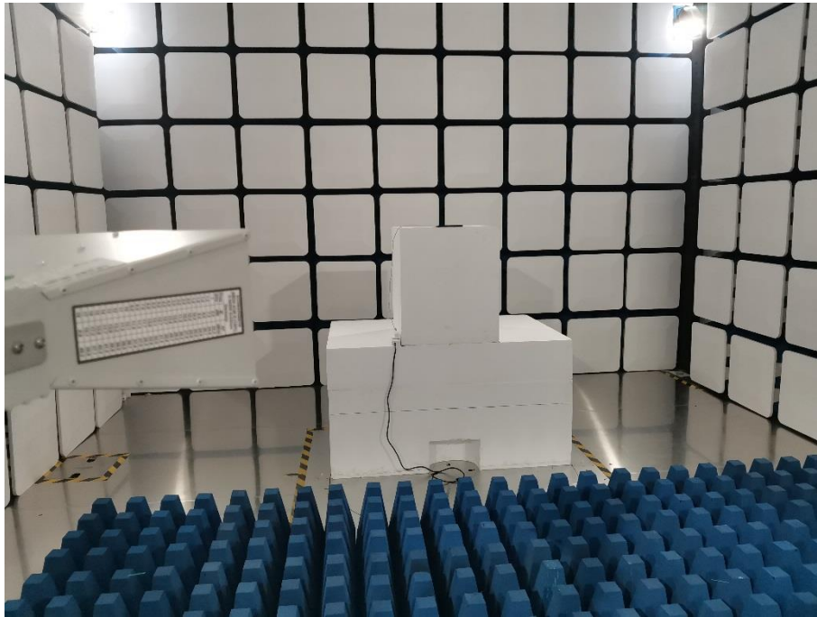
Above 1GHz-BT/BLE/WIFI
