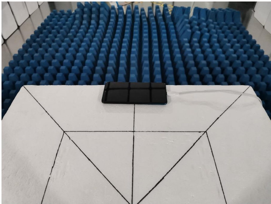
Close-Up-BT/BLE/WIFI
