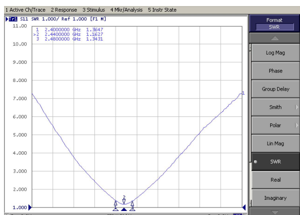
VSWR
