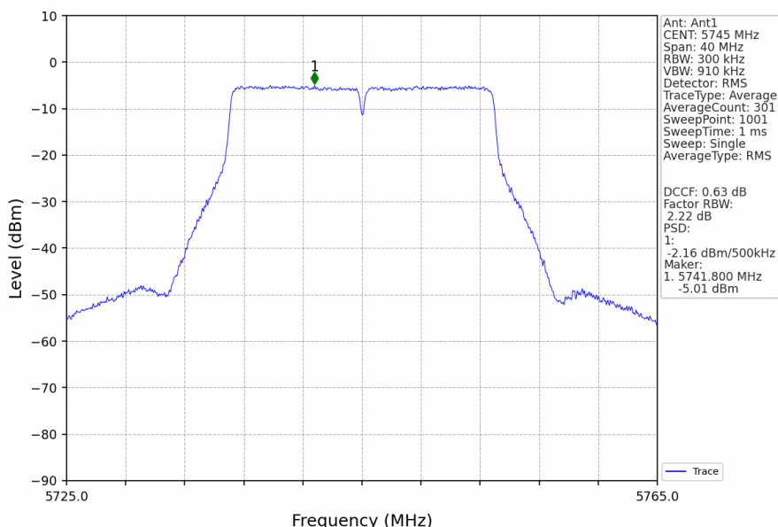
802.11n(HT20)_LCH_5745MHz_Ant1_NTNV
