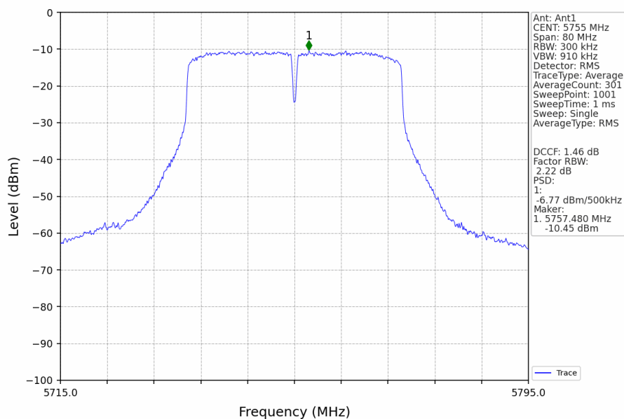
802.11ac(VHT40)_LCH_5755MHz_Ant1_NTNV
