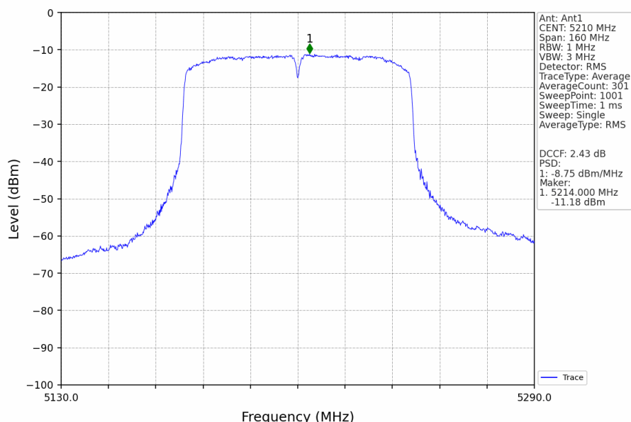
802.11ac(VHT80)_MCH_5210MHz_Ant1_NTNV
