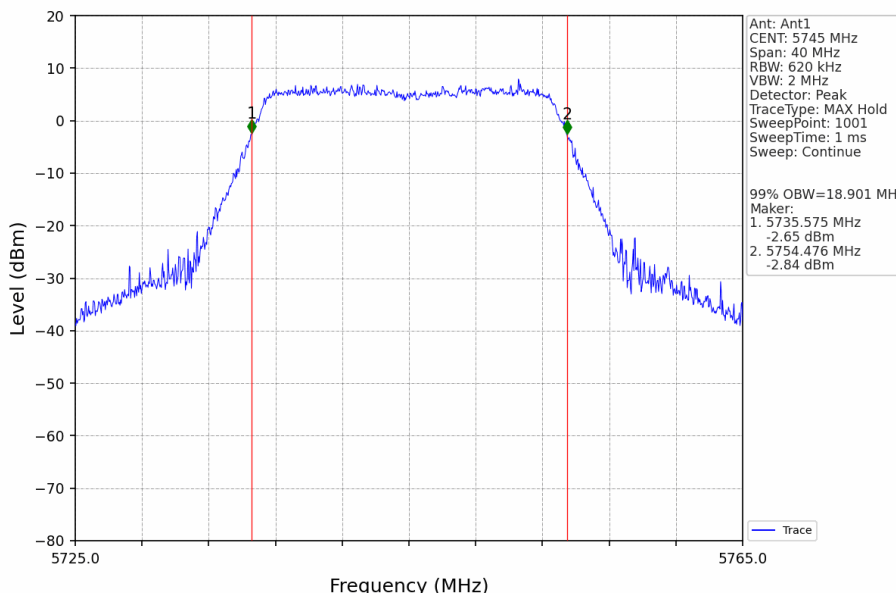
802.11n(HT20)_LCH_5745MHz_Ant1_NTNV
