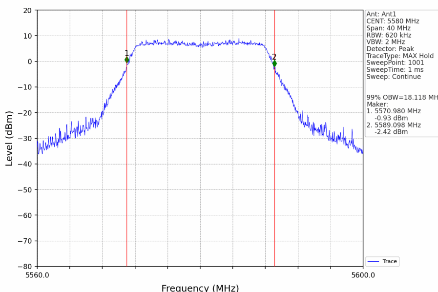
802.11a_MCH_5580MHz_Ant1_NTNV
