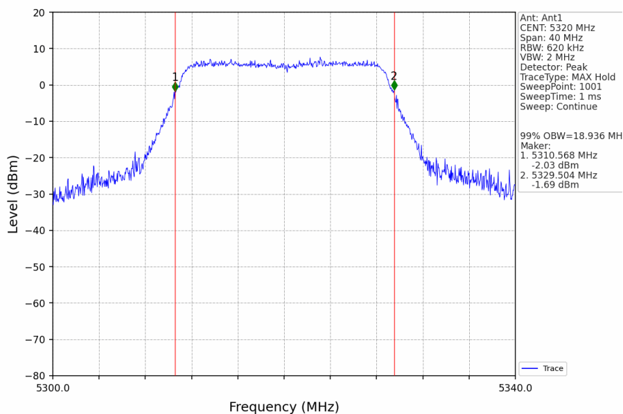
802.11n(HT20)_HCH_5320MHz_Ant1_NTNV
